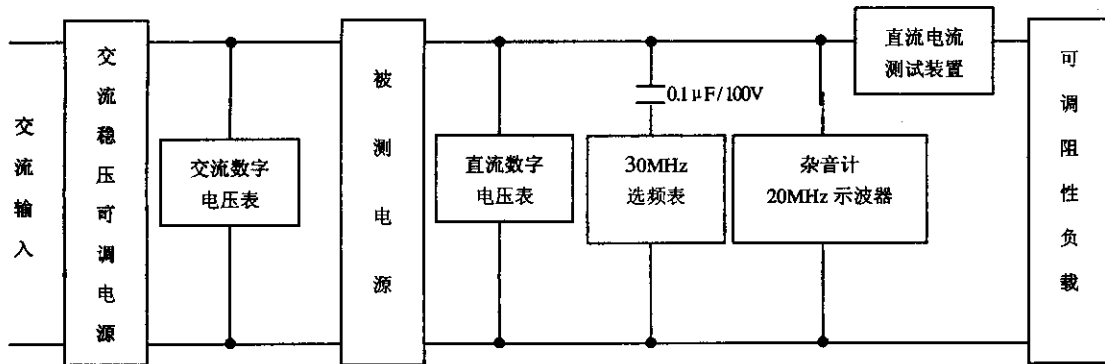
图2 杂音电压试验电路
