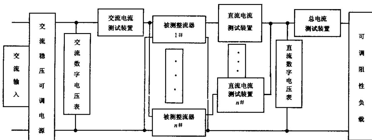
图4 均分负载性能试验电路
