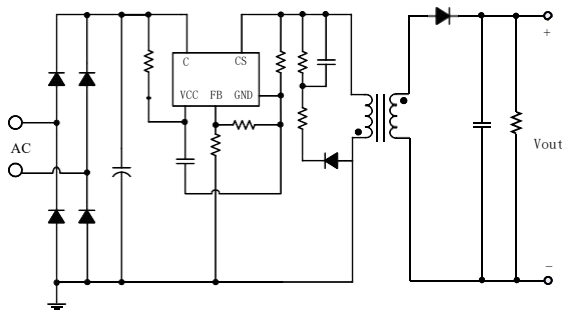
图 1 ICW4009 双绕组典型应用
