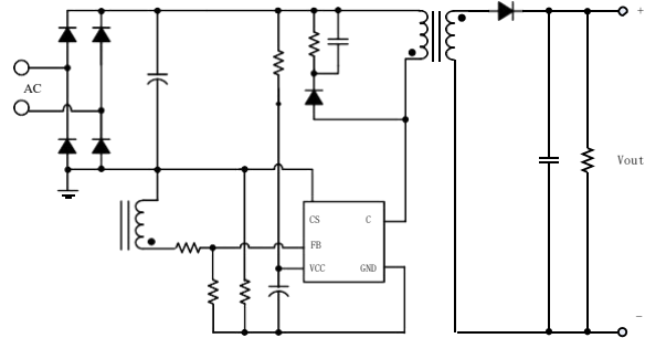
图 2 ICW4009 三绕组典型应用
