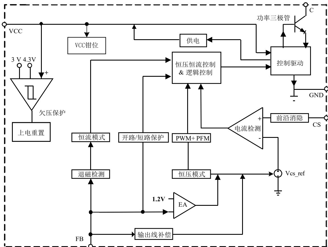
图 4 ICW4009 内部框图
