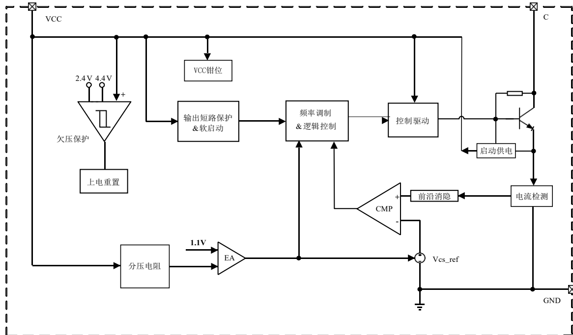
图3 ICW4007 内部框图
