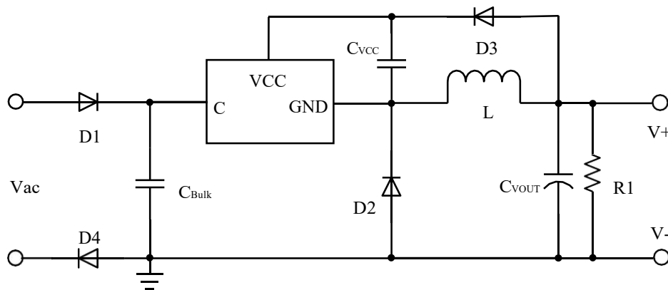
图 1 ICW4007 Buck 典型应用
