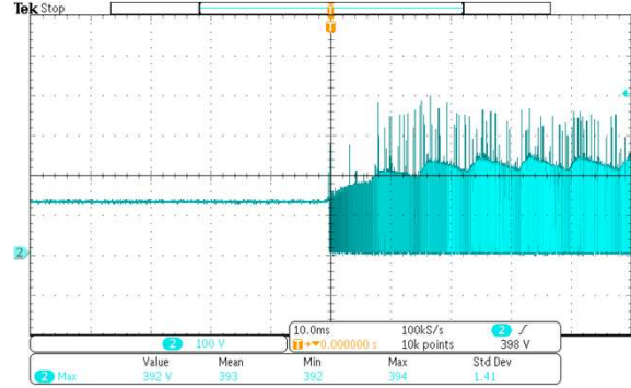
90Vac Turn On Vds(max) : 392V
