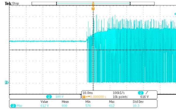
264Vac Turn On Vds(max) : 612V
