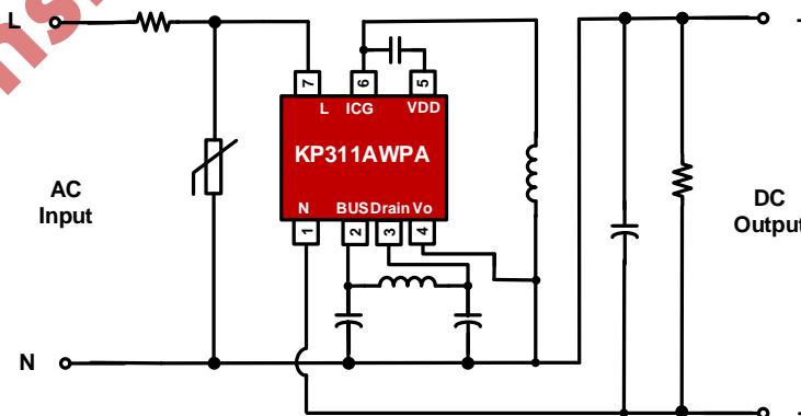
图 1 典型应用电路图
