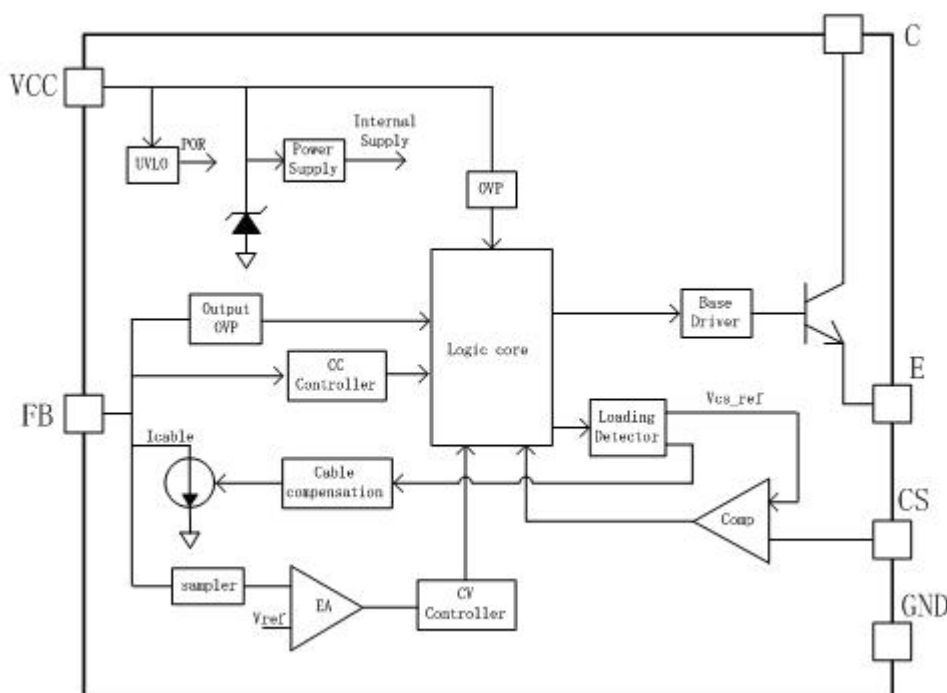
图 3 S710x 内部结构框图
