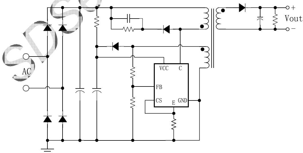
图1 S710x 典型应用
