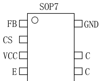
图2 脚位图
