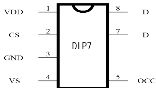
Fig3. 引脚定义(芯片无 PIN6 引脚, 标示 8 脚仅为便于理解)
