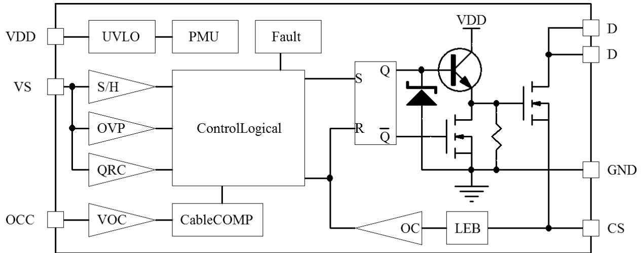
Fig2. 内部框图
