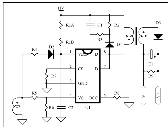
Fig1. 典型连接图
