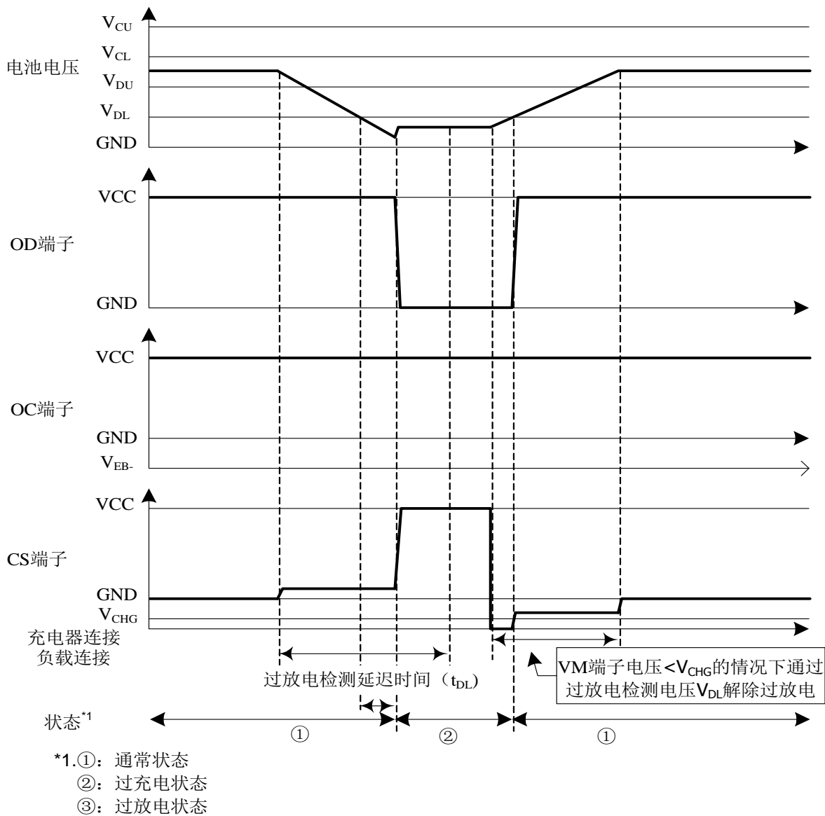
图 5. 充电器检测
