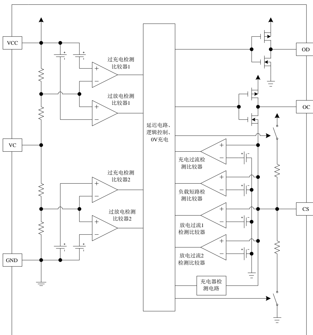
图 2. 功能框图
