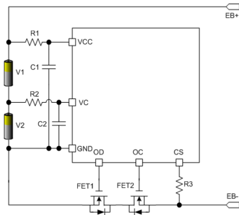
图 6. ZCC2122 典型应用电路
