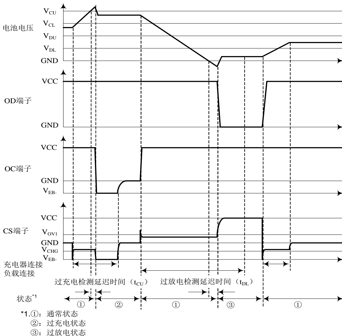
图 3. 过充电检测、过放电检测
