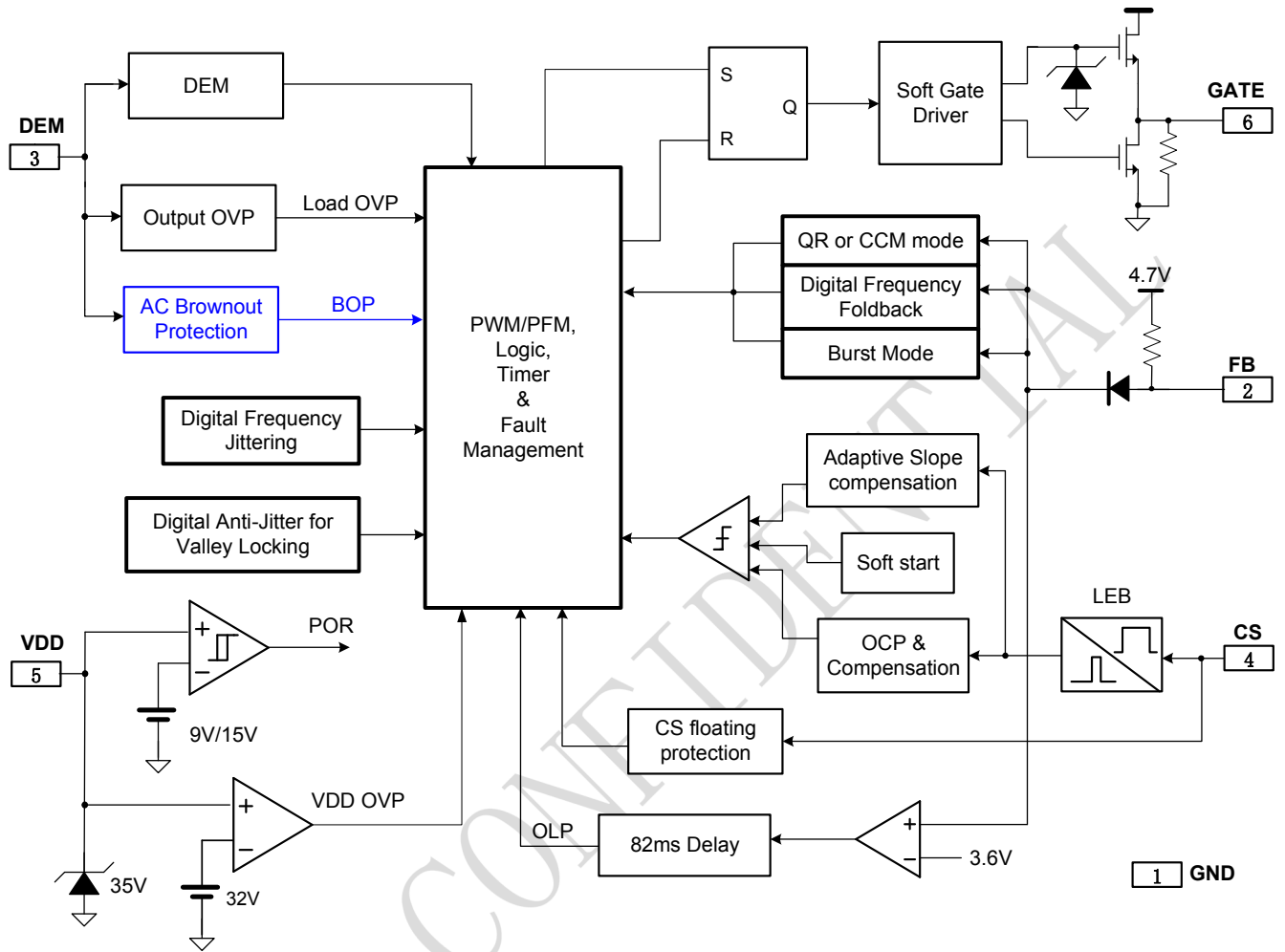
图 3 LP8773 内部框图
