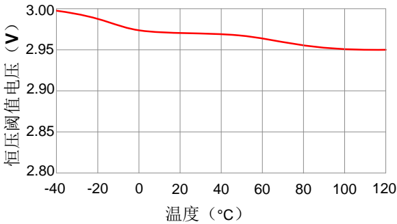
恒压阈值和温度关系
