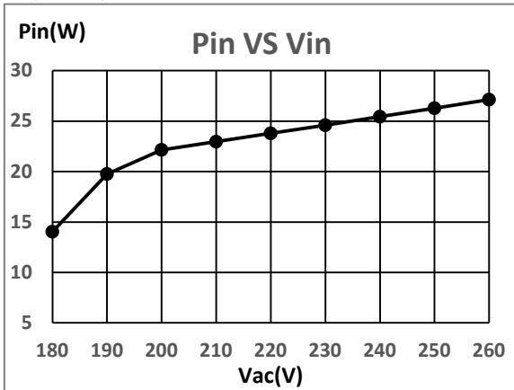
功率 VS 市电
