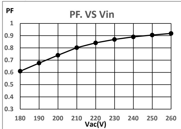
PF vs 市电
