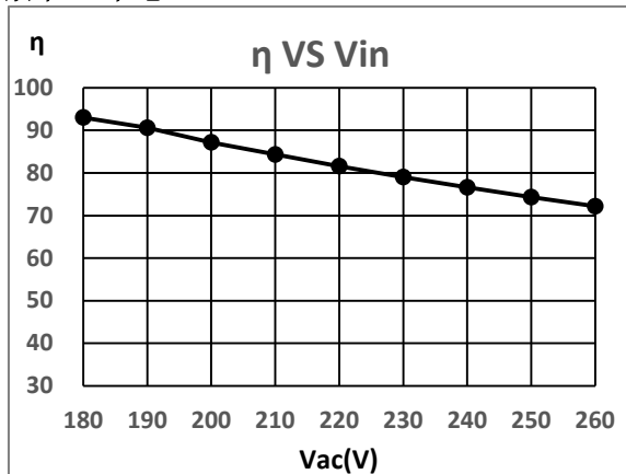
效率 vs 市电
