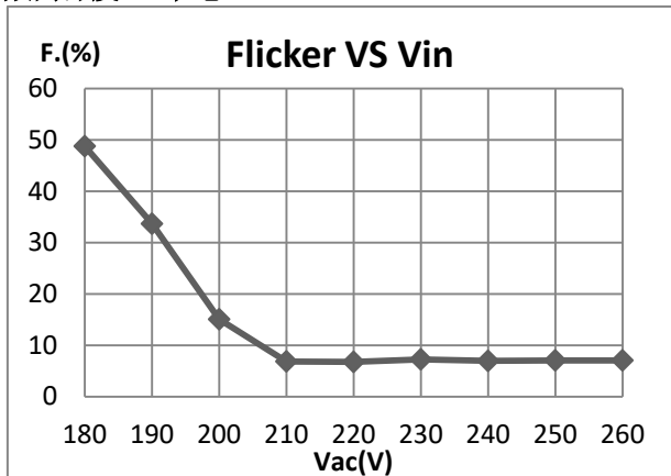
频闪深度 vs 市电
