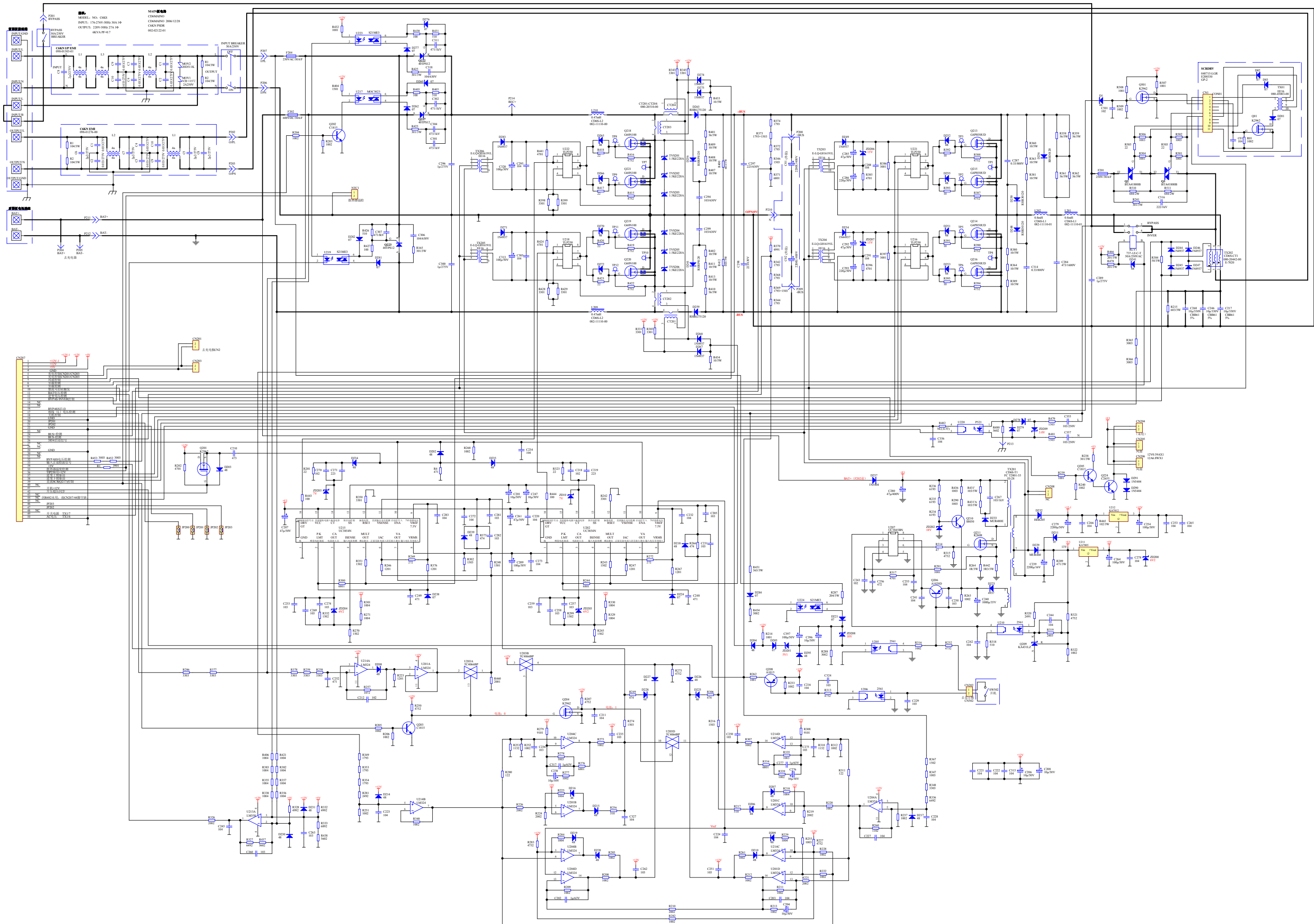
图9.1 SANTAK-C6KS型高频机主板原理图
