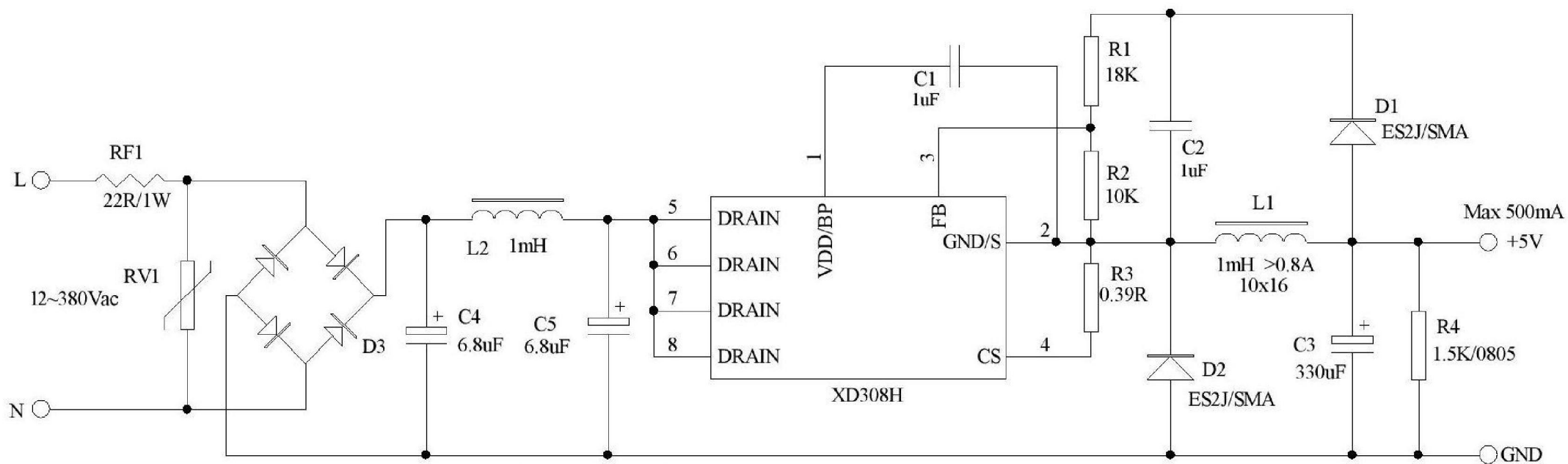
宽电压交流输入:12~380Vac; 直流稳压输出5V/500mA 的非隔离电源电路原理图
