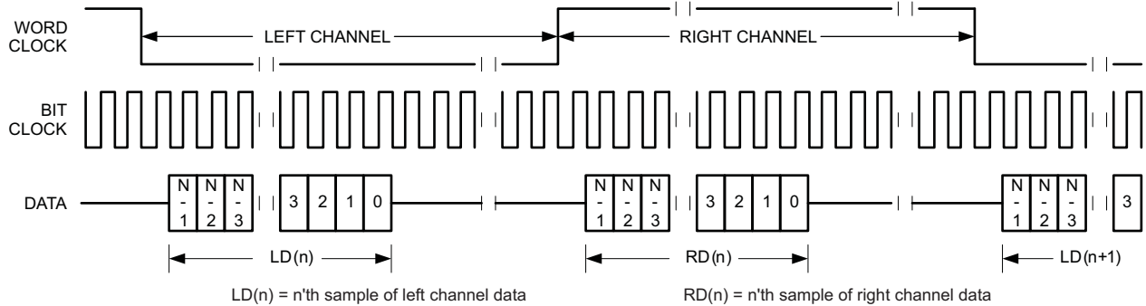
图 27. Timing Diagram for I 2 S Mode
