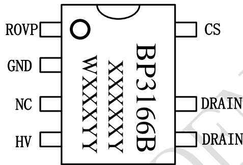
图 2 管脚封装图
