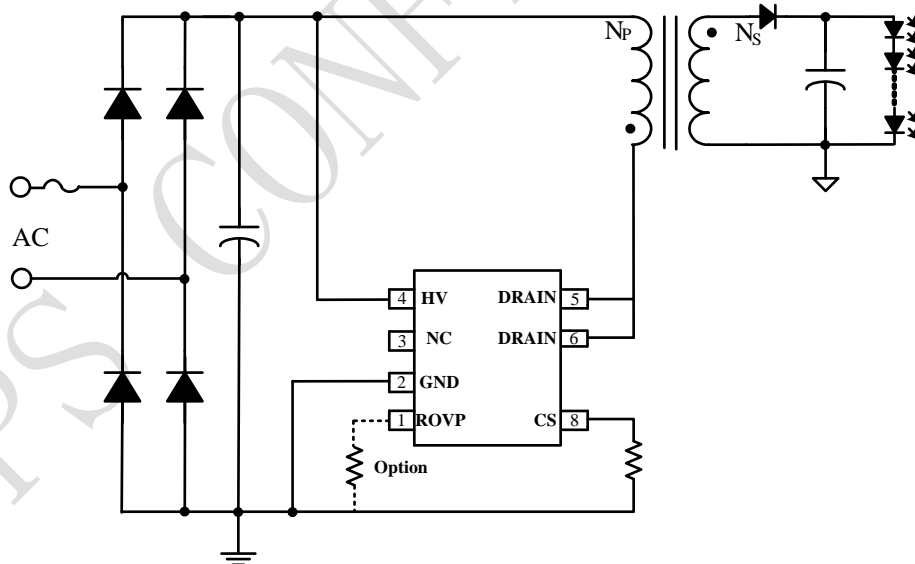
图 1 BP3166B 典型应用图
