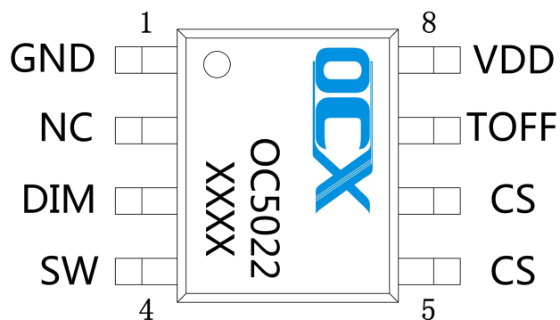
ESOP8
