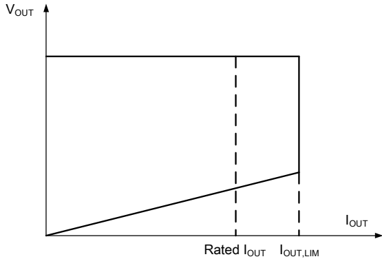
Fig. 6 V-I curve
