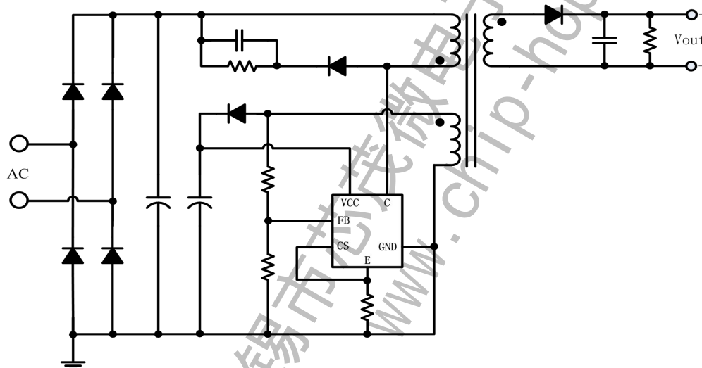
图 1 LP3783 典型应用图
