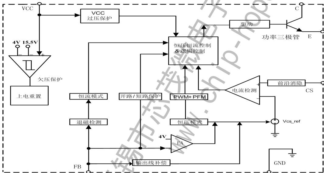
图 3: LP3783 内部框图
