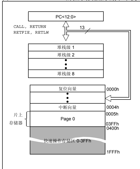
图 2-1: PIC16F631 的程序存储器映射和堆栈
