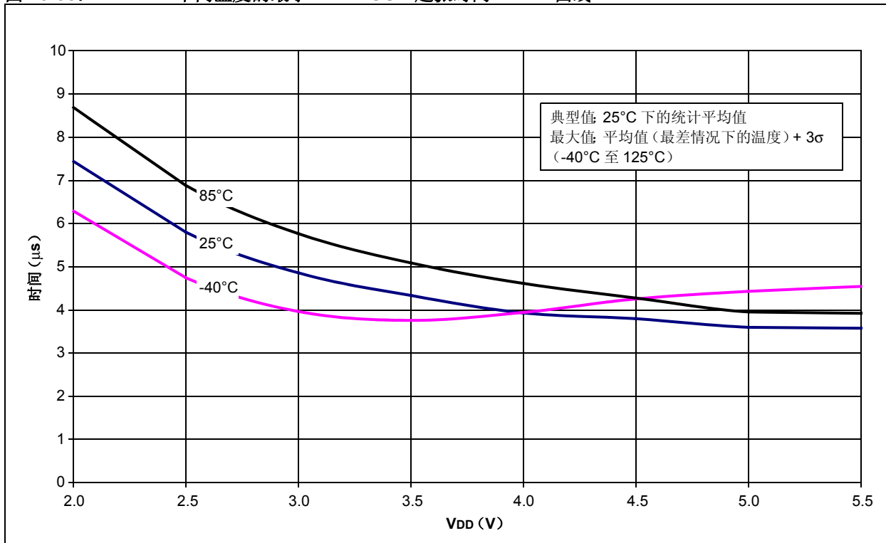
图 18-38: 不同温度的最小 HFINTOSC 起振时间 - VDD 曲线
