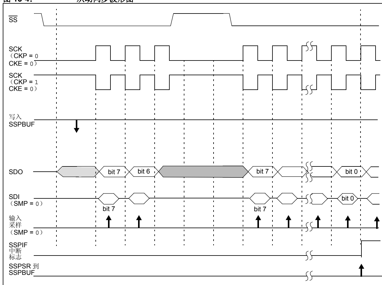
图 13-4: 从动同步波形图
