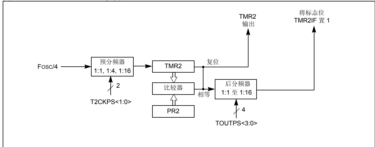
图 7-1: TIMER2 框图
