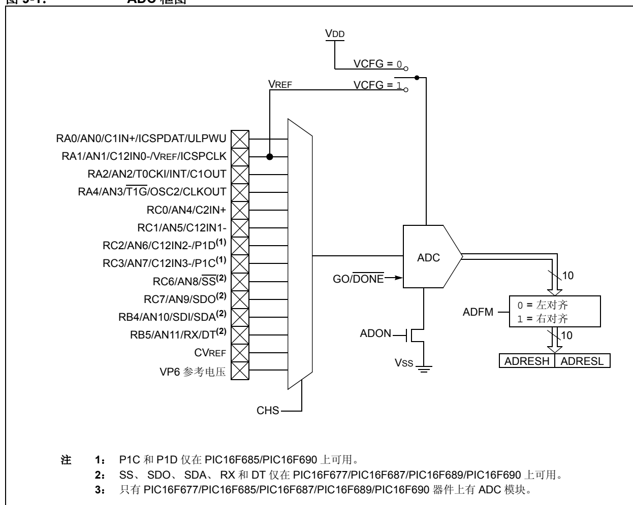
图 9-1: ADC 框图
