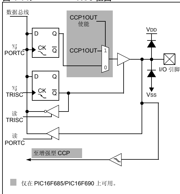
图 4-14: RC5 框图
