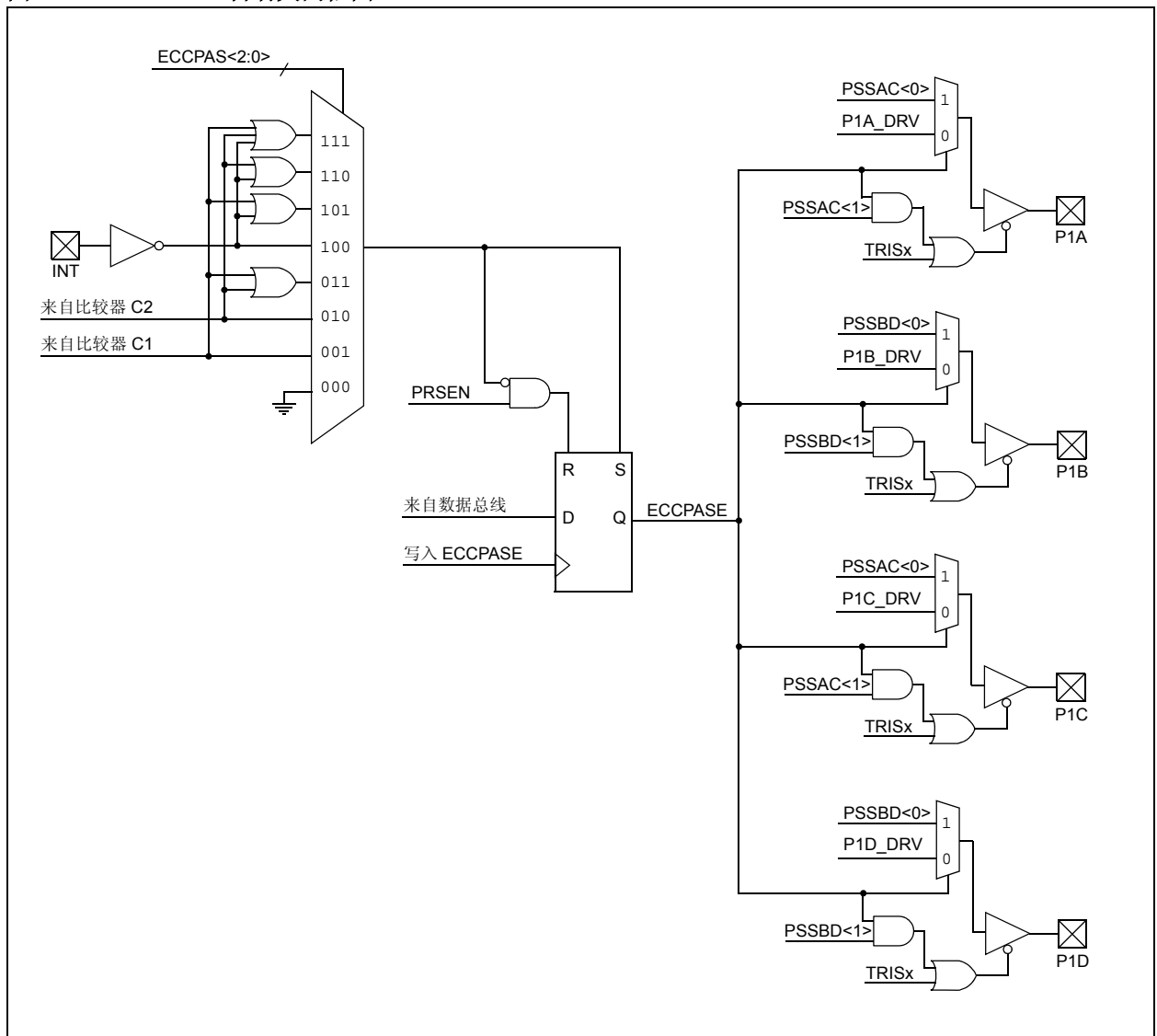
图 11-14: 自动关闭框图
