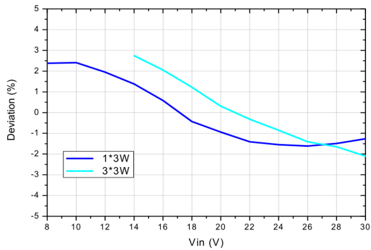
(5) 3W LED 灯输出电流变化率与输入电压关系:
