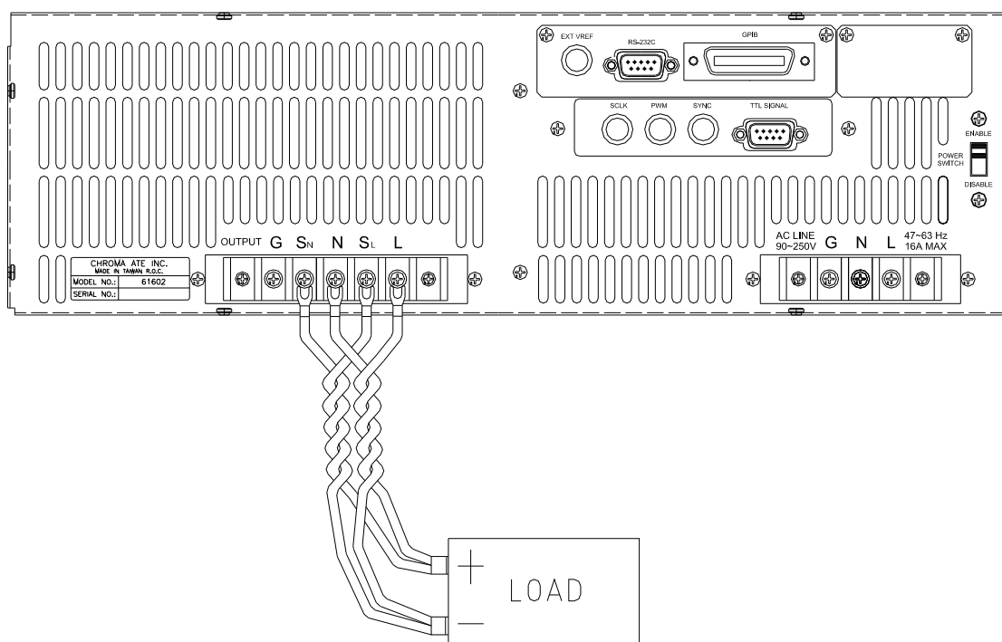
圖 2-3 輸出 & 遙測連接
