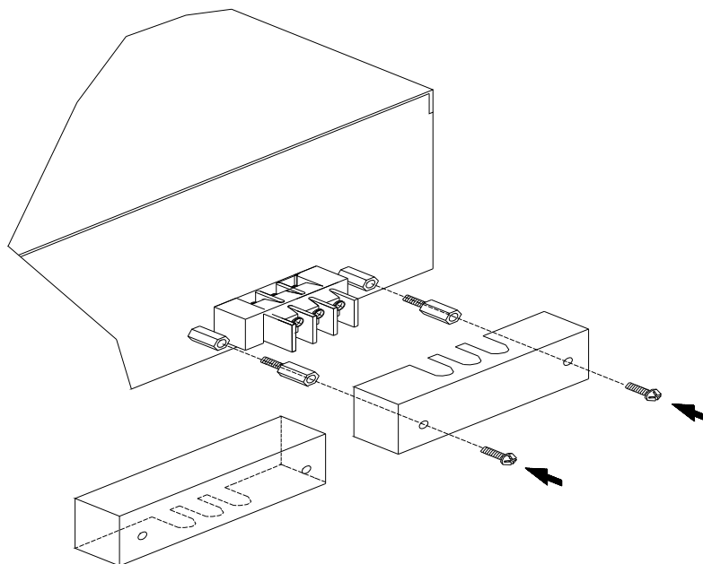
圖 2-2 輸入端子外殼
