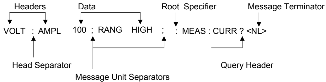
圖 7-1 指令訊息的結構
