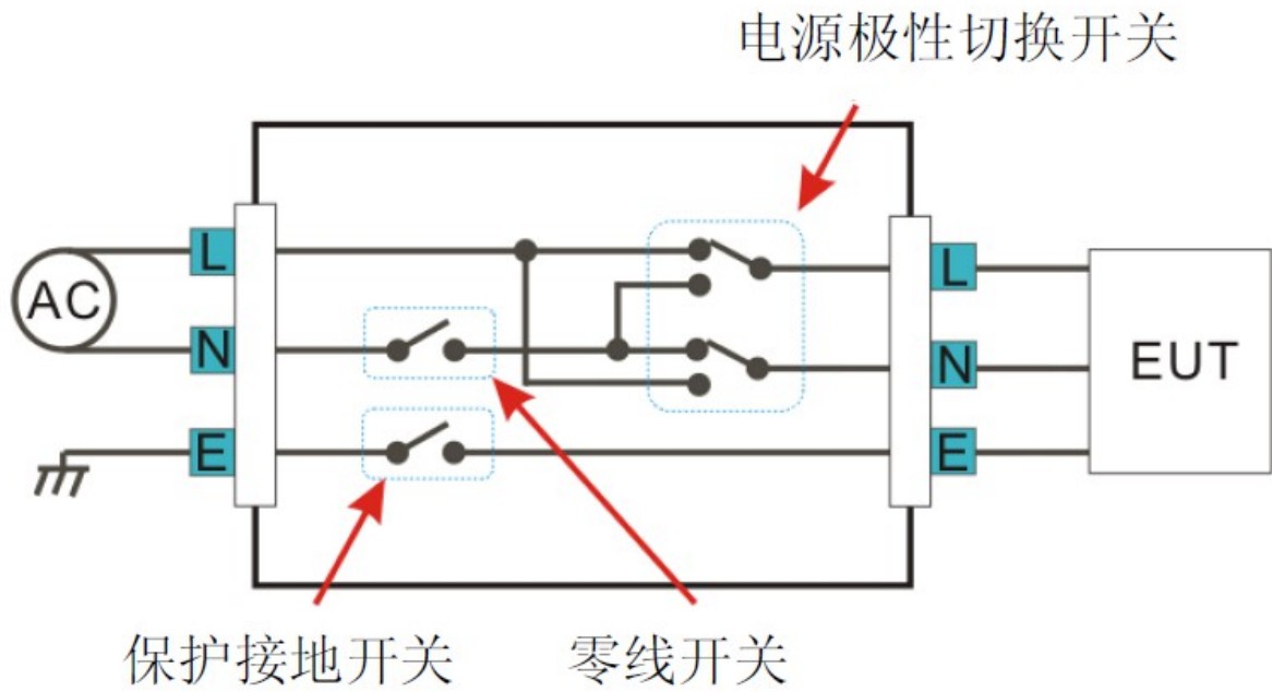
GLC-9000 测试示意图
