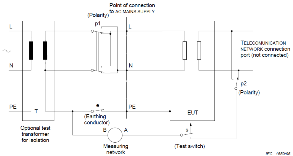
上图是 IEC60990 标准里面的连线测试图
