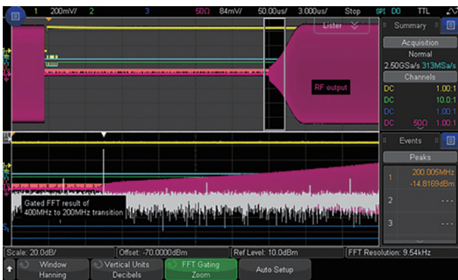
图 21c: 开始发现在 200MHz 上的射频信号。您也能通过射频模拟波形进行验证
