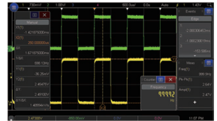
图 3: 侧边栏配有可移动的测量/分析窗口,支持您将窗口放置在屏幕的任何位置
