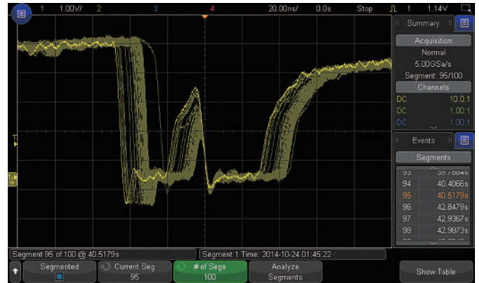
图13a: 屏幕显示了100个分段的包络图, 可进行最坏情况的波形分析
