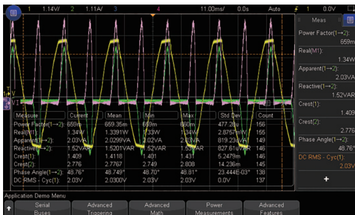
图 29: 集成的功率测量可以让您快速分析电源和功耗器件。
