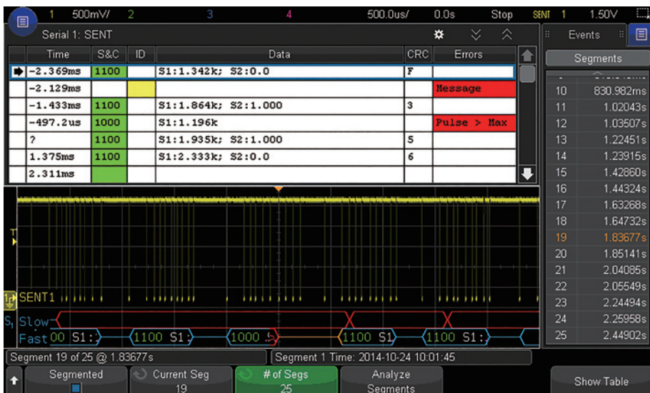
图 20: 分段存储器与串行解码配合使用, 能够对串行总线进行最深入的分析。
