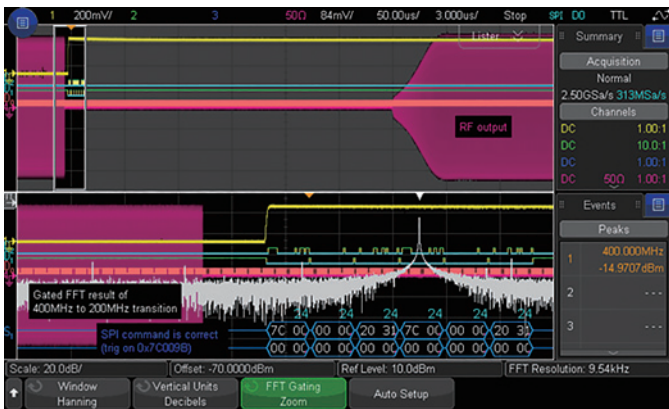
图 21a: 在 SPI 命令上触发时，射频信号的频率仍然是 400 MHz，如列表显示器中的频率峰值搜索结果所示
