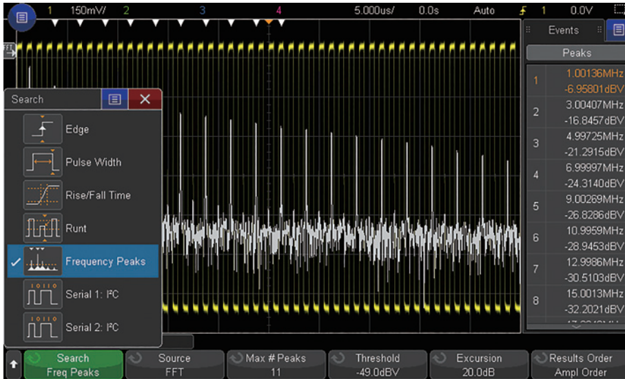
图 14: 把 3000T X 系列设置为捕获用于 FFT 分析的时钟信号。使用搜索和导航功能，示波器能够查找、标记(白色三角形)并快速导航到最先出现的 11 个频率峰值。您可以按照频率或幅度的次序进行排序。
