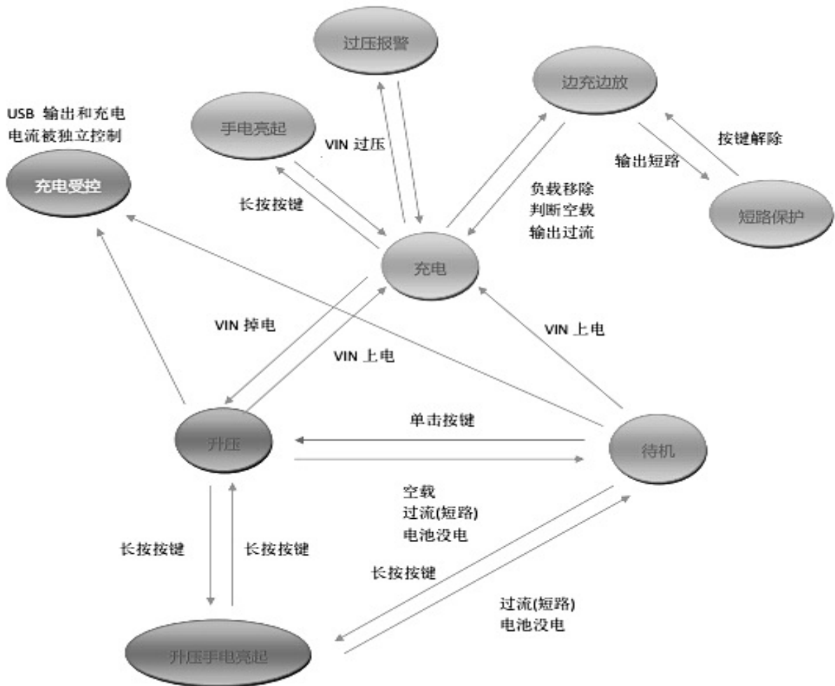
ZS6599 状态转换图
