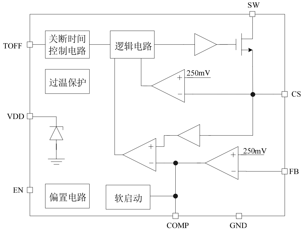
图 2：6702 的内部电路方框图
