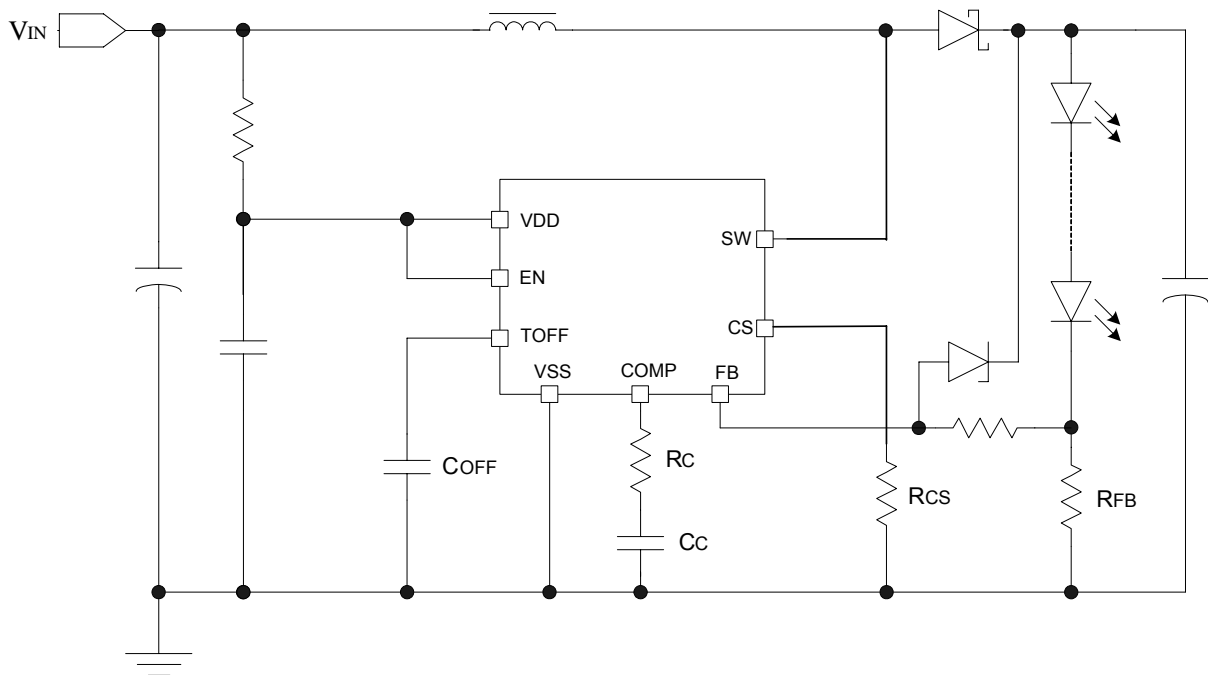
图 1：6702 典型应用电路图
