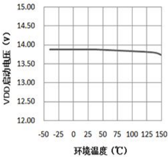
VDD 启动电压对温度的变化
