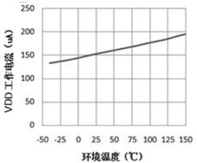
VDD 工作电流对温度的变化
