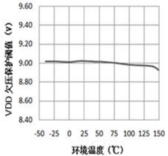
VDD 欠压保护阈值对温度的变化
