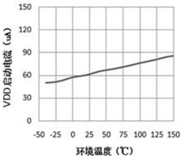
VDD 启动电流对温度的变化
