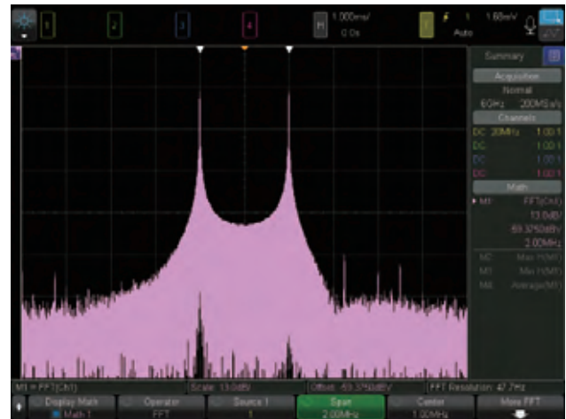
图36. 传统的单色FFT功能有限。
