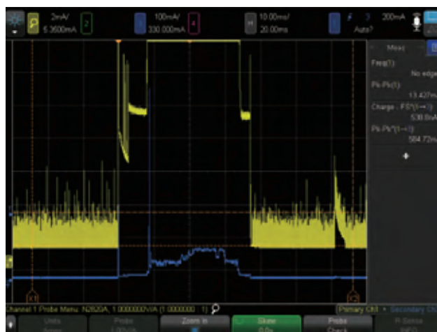
图55. 手机待机和工作状态时的电流消耗放大和缩小视图。
