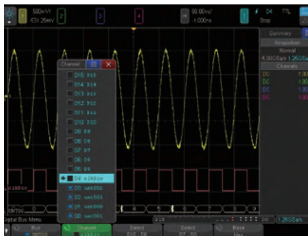
图 46. FPGA 动态探头屏幕截图
