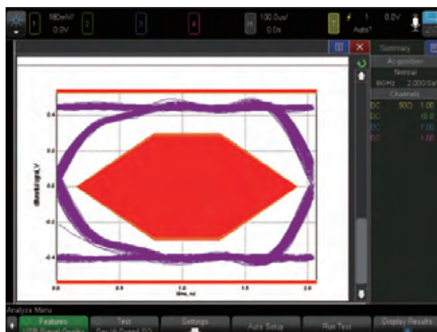
图44. USB 2.0高速近端眼图测试
