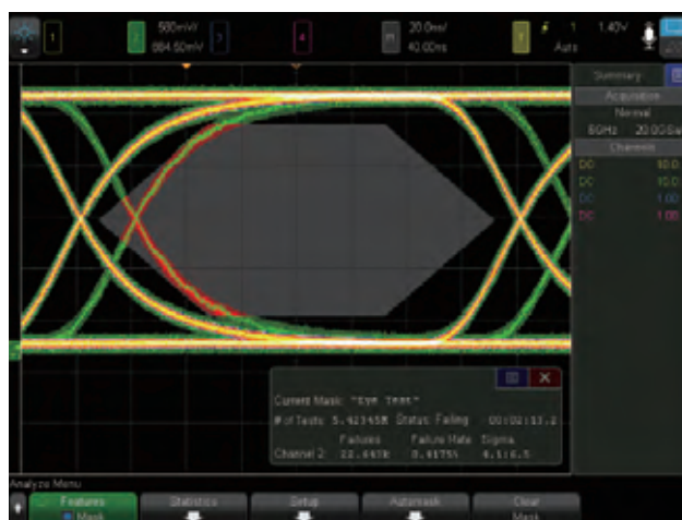
图41. 串行数据模板测试
