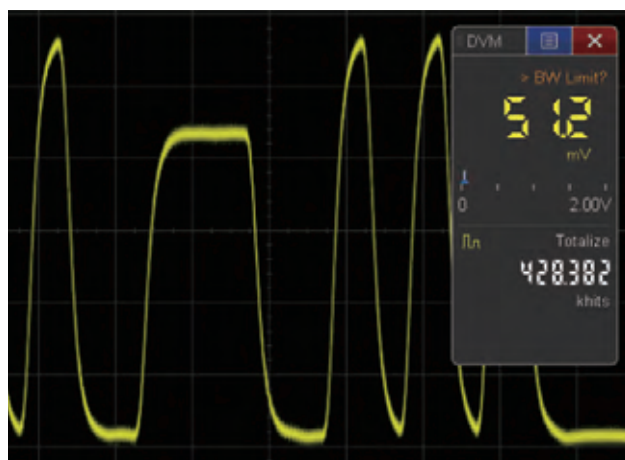
图 35. 计数矮脉冲的总数
