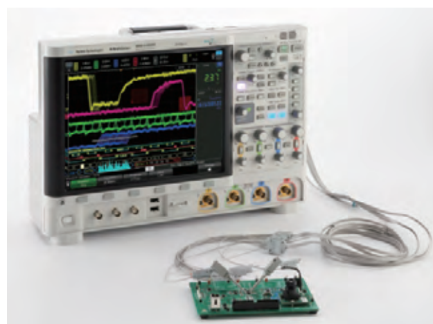
图27. MSO配有新型逻辑通道探头
