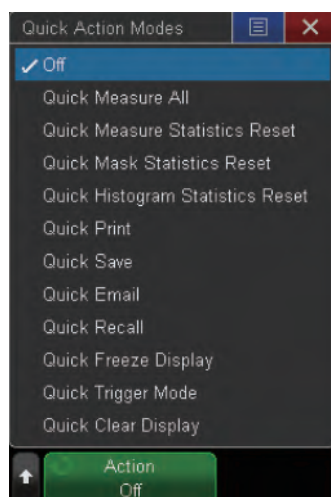
图 56. QuickAction 菜单
