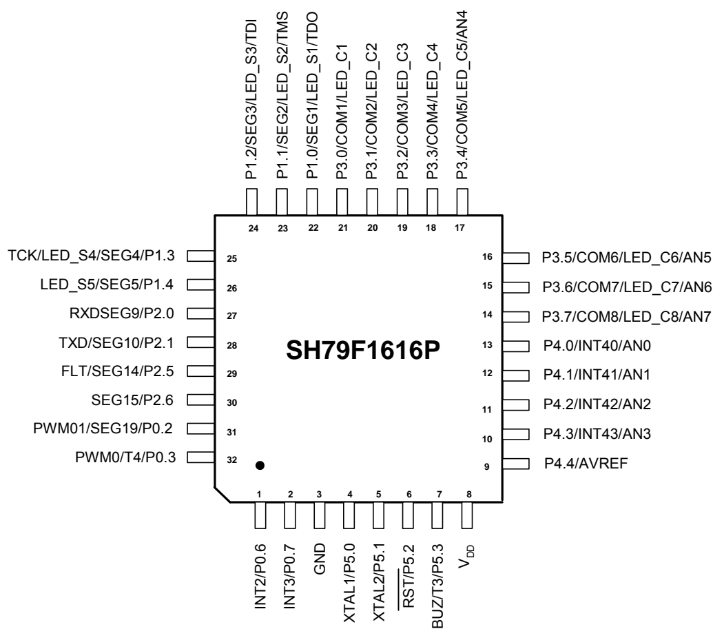
LQFP32 引脚配置图
