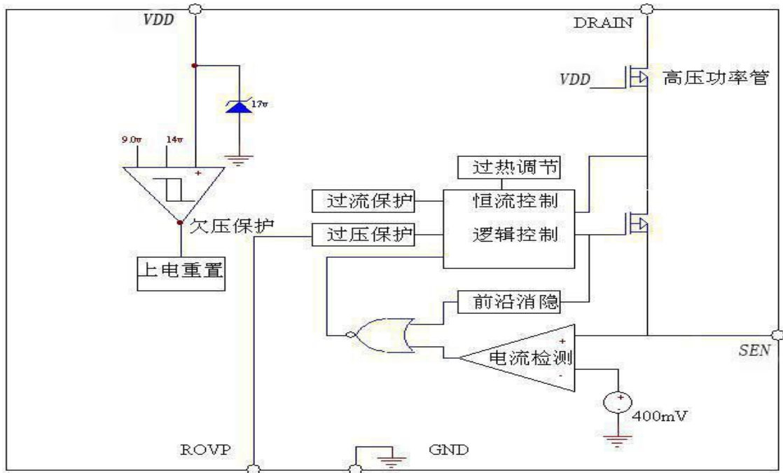
图 3 M8833 内部框图
