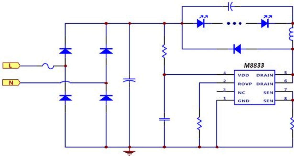
图 1 M8833 典型应用图
