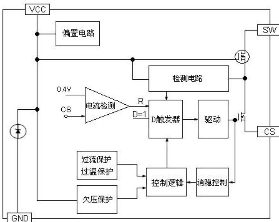
图二，OCP8160 内部方块电路图
