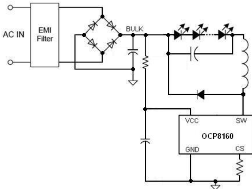
图一， OCP8160 典型应用电路
