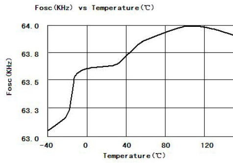
Figure 6.4 Fosc(KHz) vs Temperature(°C)
