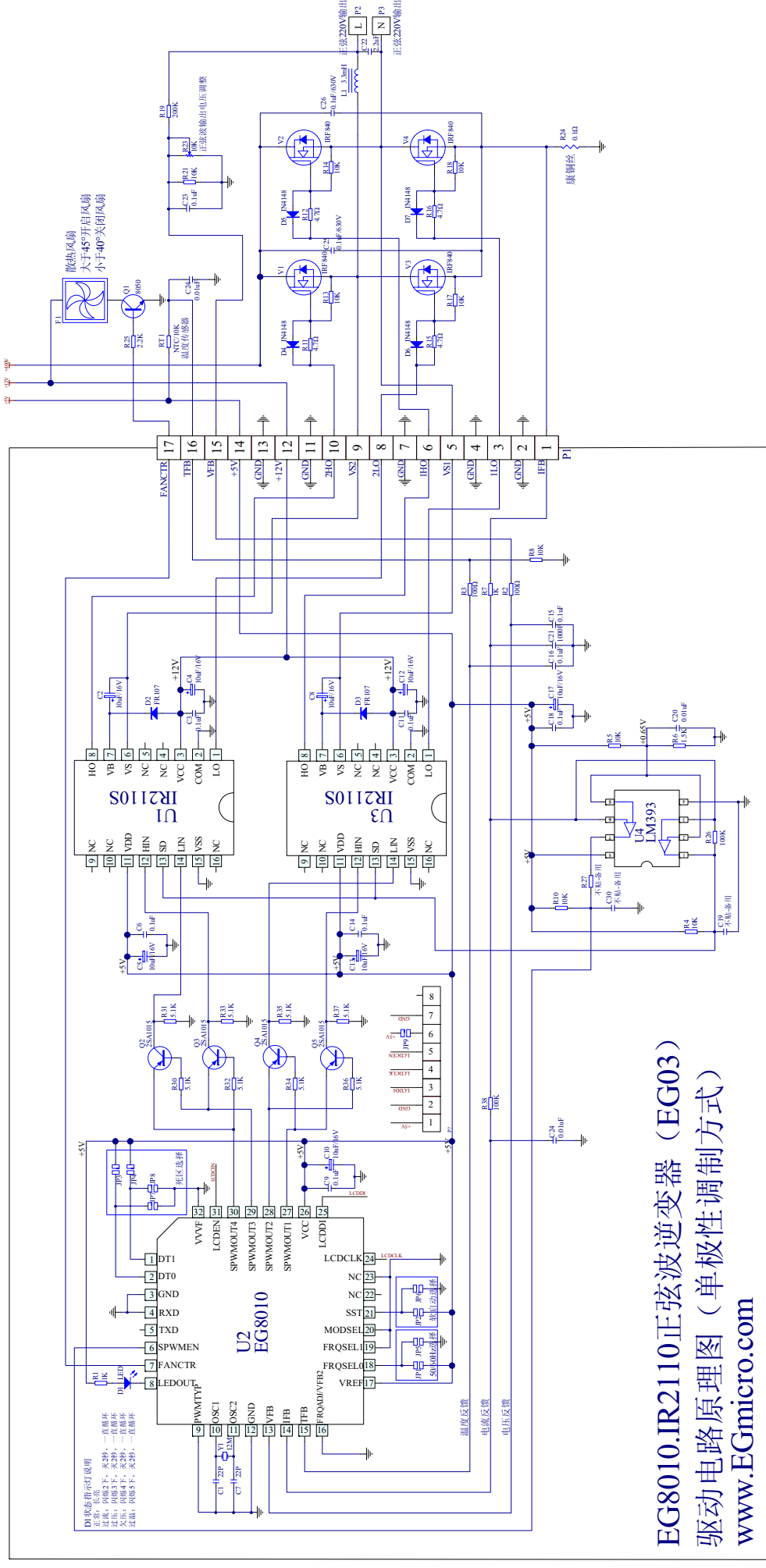
图 6-2. EG8010+IR2110S+闭锁纯正弦波逆变器典型应用电路图 (单极性调制方式)
