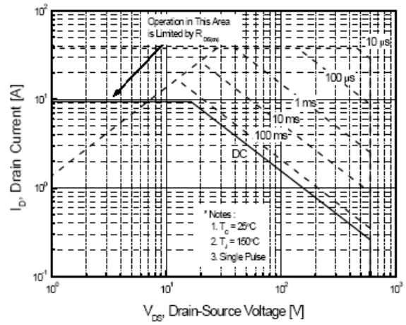
图 6-2 CR12N65C(TO-220FP) 最大安全工作区曲线
