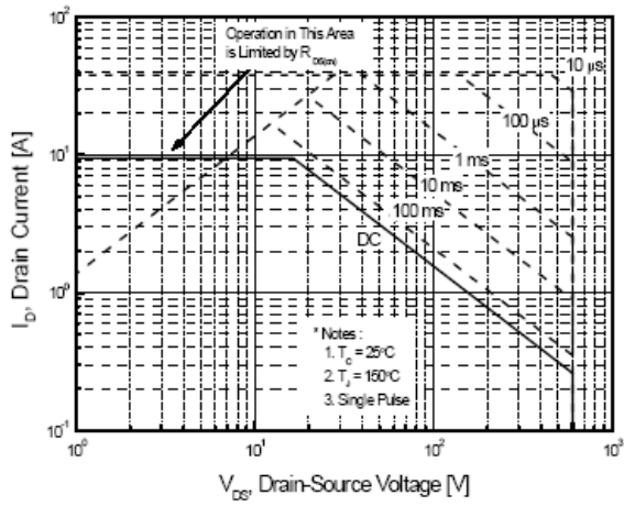
图 6-1 CR12N65C(TO-220) 最大安全工作区曲线
