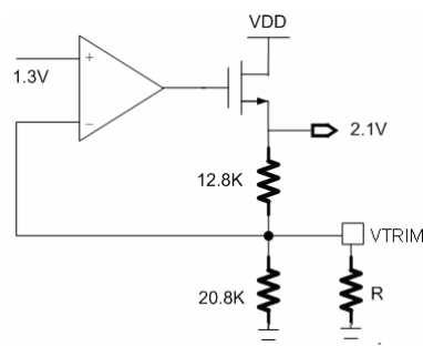
图 3. 充饱电压调整示意图
