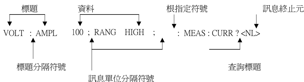
圖 6-1 命令訊息的架構
