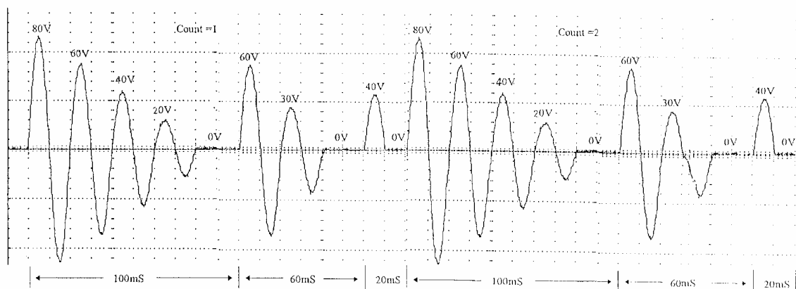
圖 3-2 LIST 暫態
