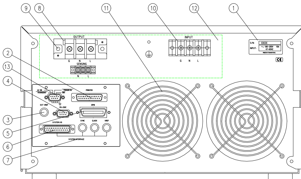
圖 1-2 後背板
