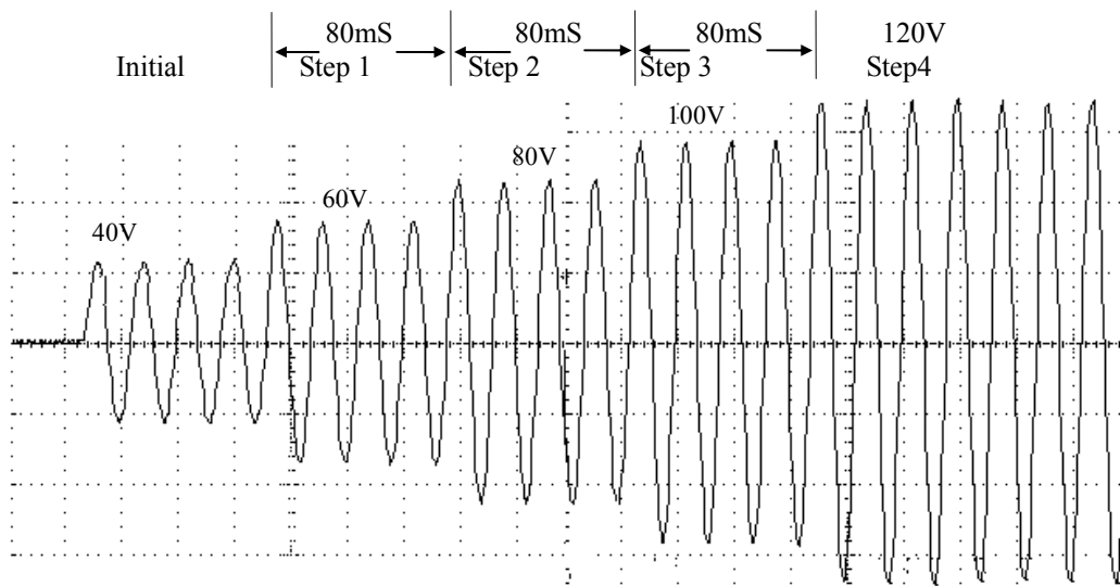
圖 3-1 STEP 暫態
