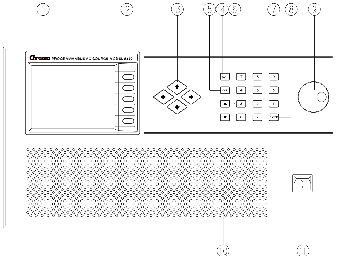
圖 1-1 前面板
