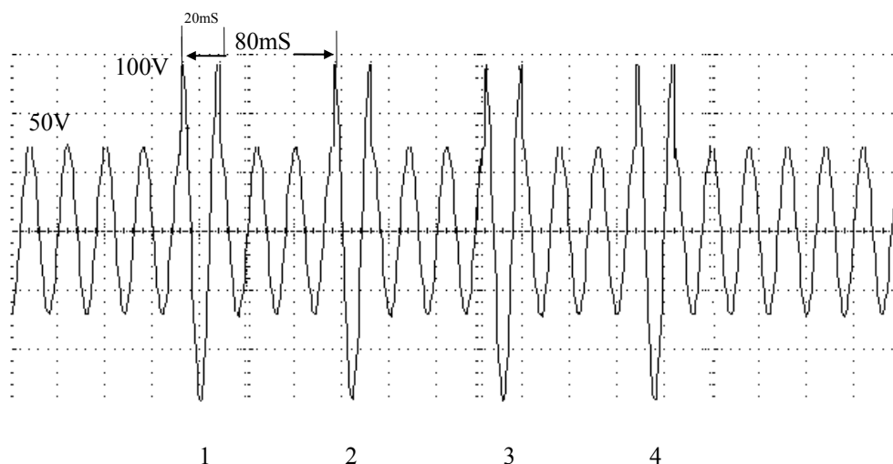
圖 3-3 PULSE 暫態
