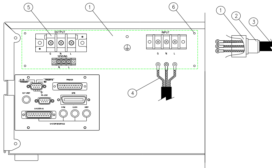
圖 2-1 連接輸入
