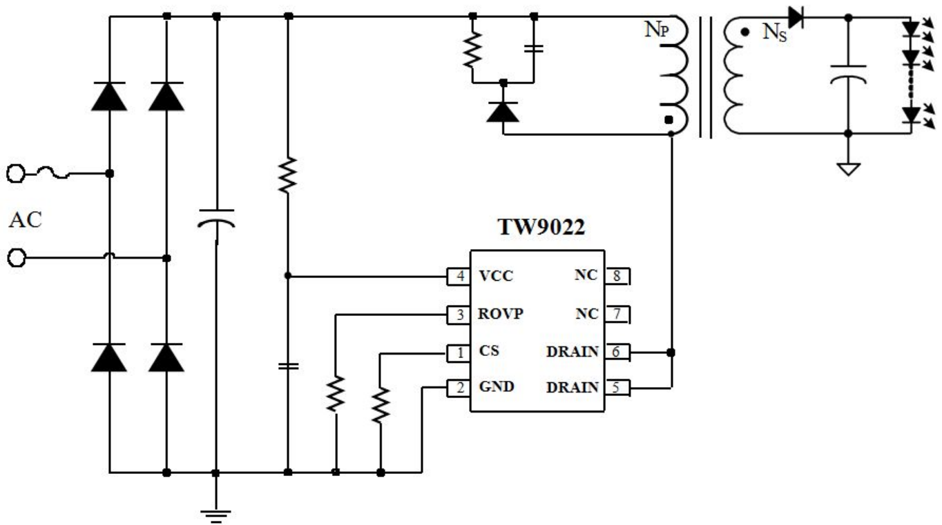
图3 TW9022典型应用图
