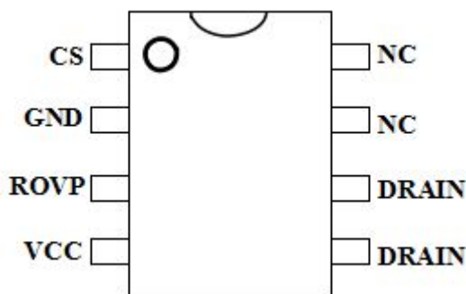
图1 管脚封装图
