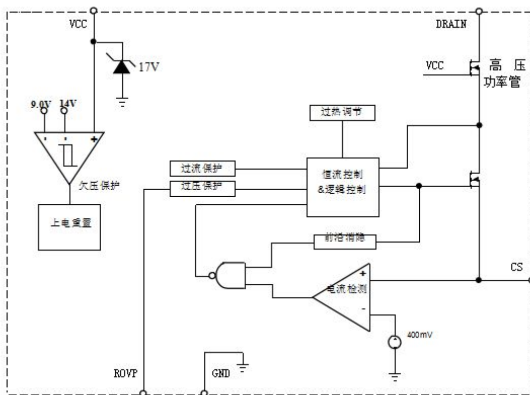
图2 TW9022内部框图
