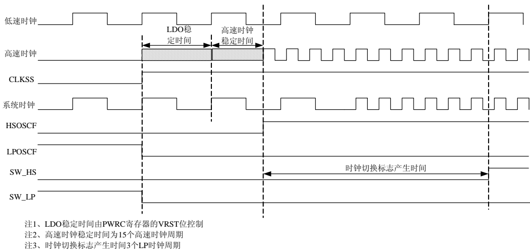
图 6-6 低速 LP 时钟切换到 INTOSCH 时钟
