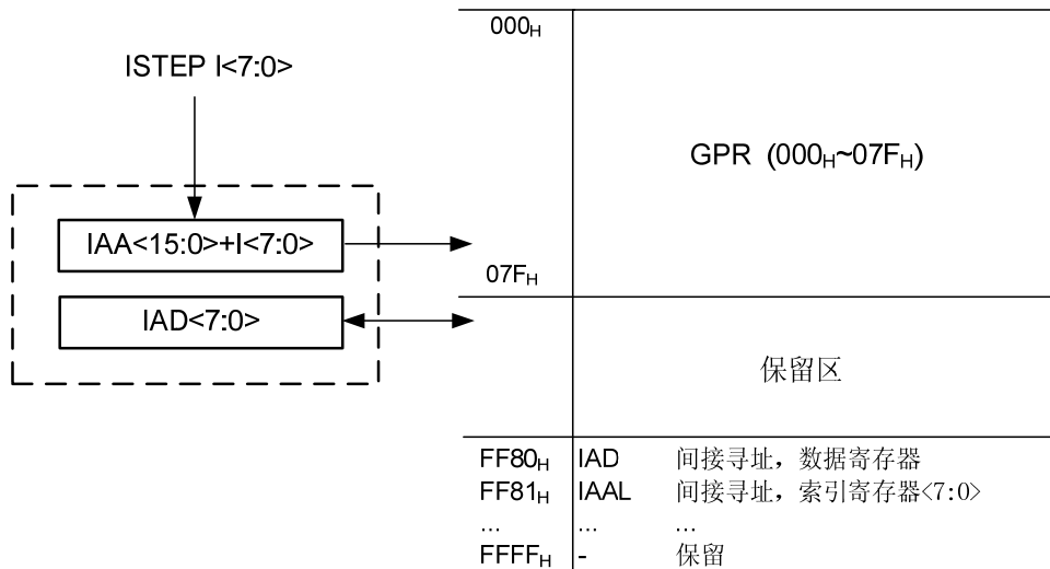
图 3-5 间接寻址示意图
