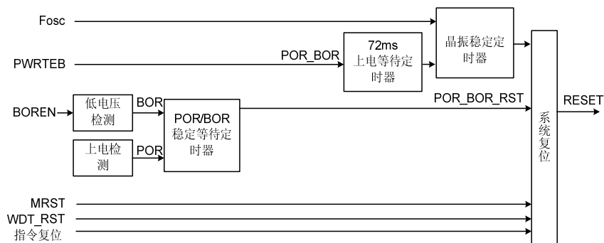
图 6-9 芯片复位原理图
