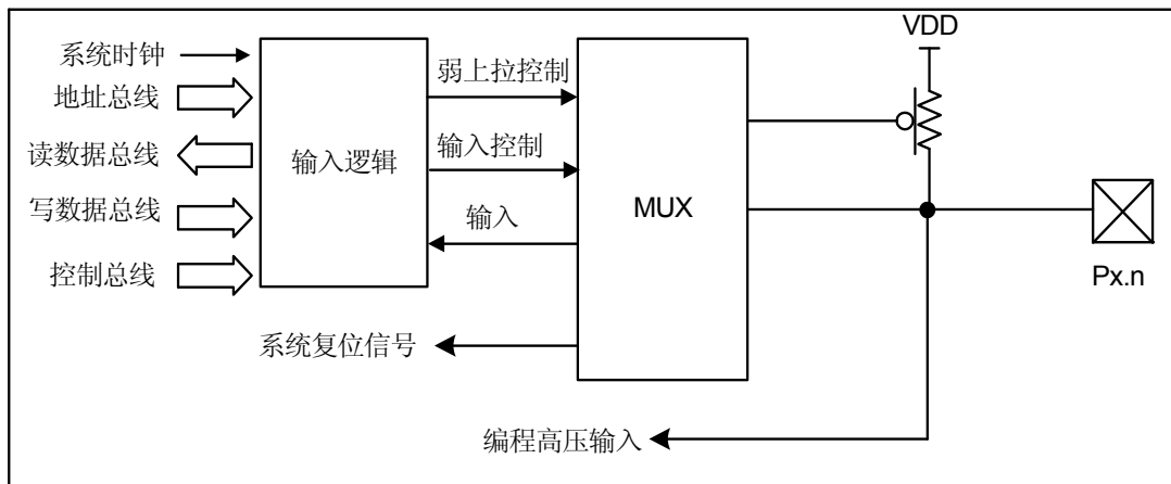
图 4-2 输入端口结构图 C
