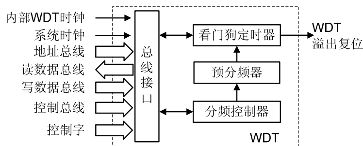
图 6-8 看门狗定时器内部结构图
