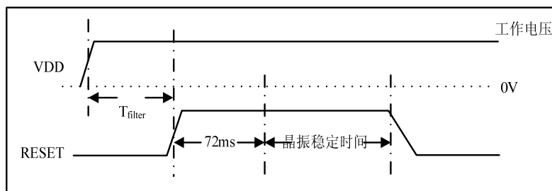
图 6-10 上电复位时序示意图
