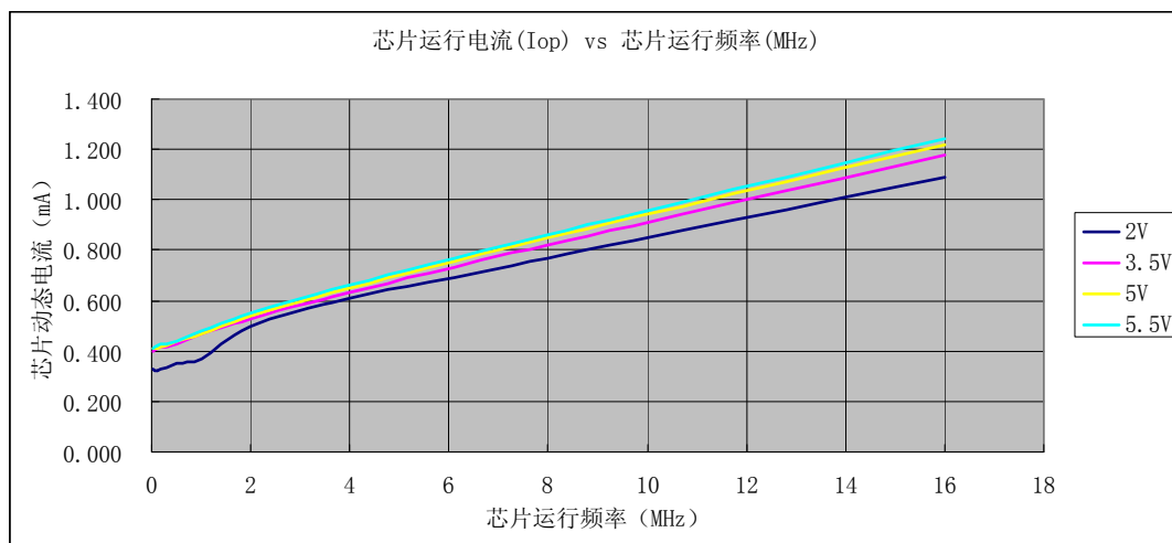
正常运行模式下芯片电流随时钟频率变化图（室温 25°C）
