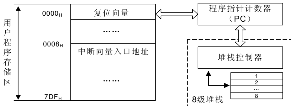
图 3-1 HR7P160 程序区地址映射和堆栈示意图
