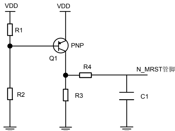
图 6-13 N_MRST 复位参考电路图 2
