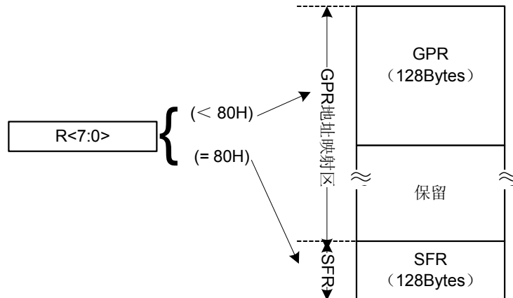
图 3-3 普通直接寻址示意图
