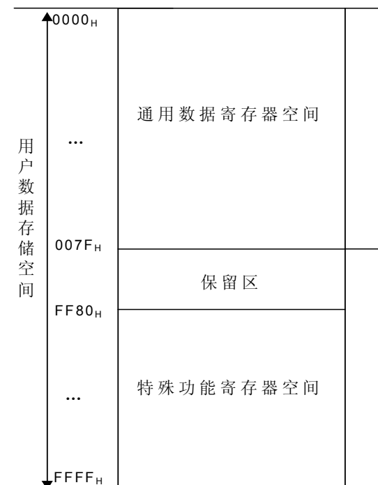
图 3-2 数据区地址映射示意图
