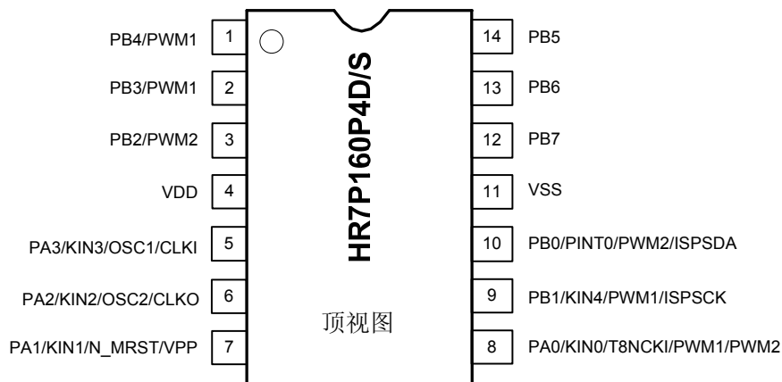
图 1-2 HR7P160P4D/S (DIP14/SOP14) 顶视图
