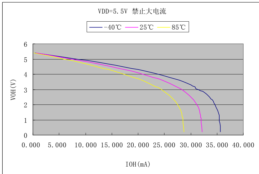
G: V_{OH} vs I_{OH} @VDD=5.5V
