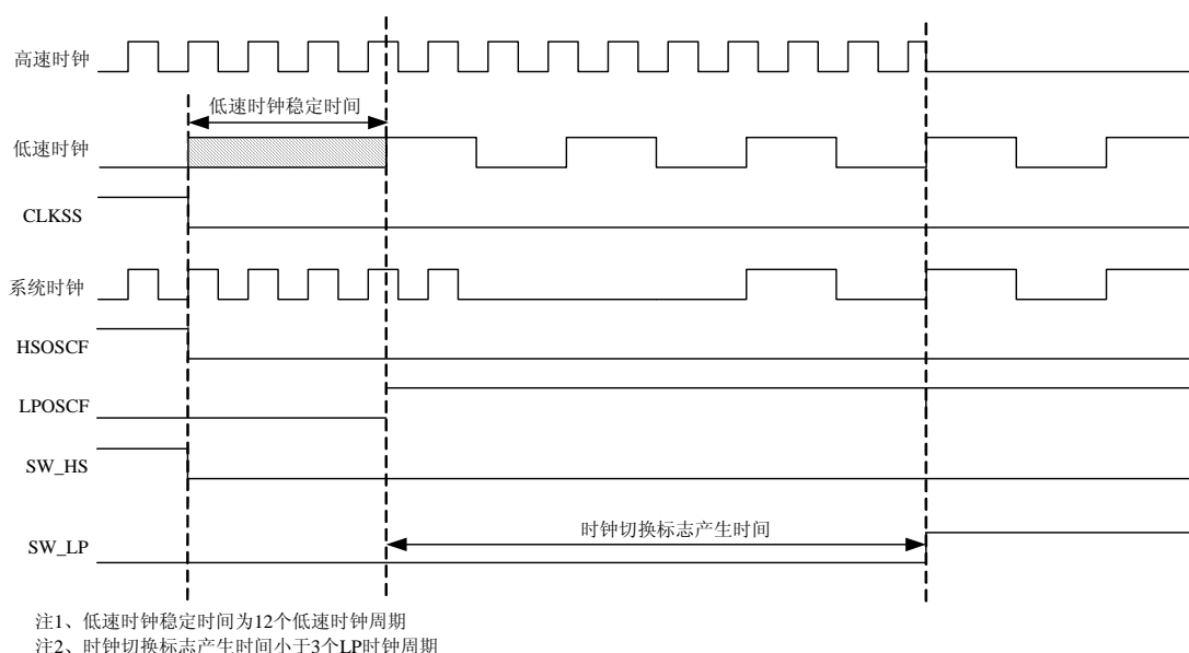
图 6-7 INTOSCH 时钟切换到低速 LP 时钟
