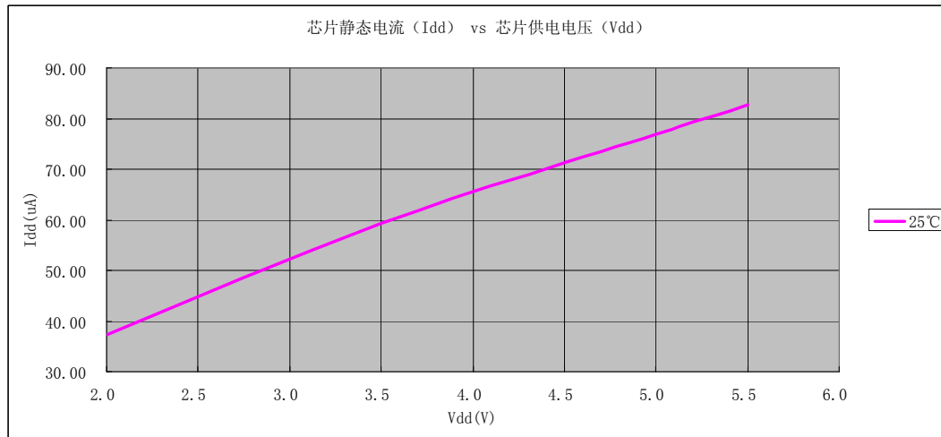
芯片静态电流随芯片电压变化特性图（室温 25°C）
