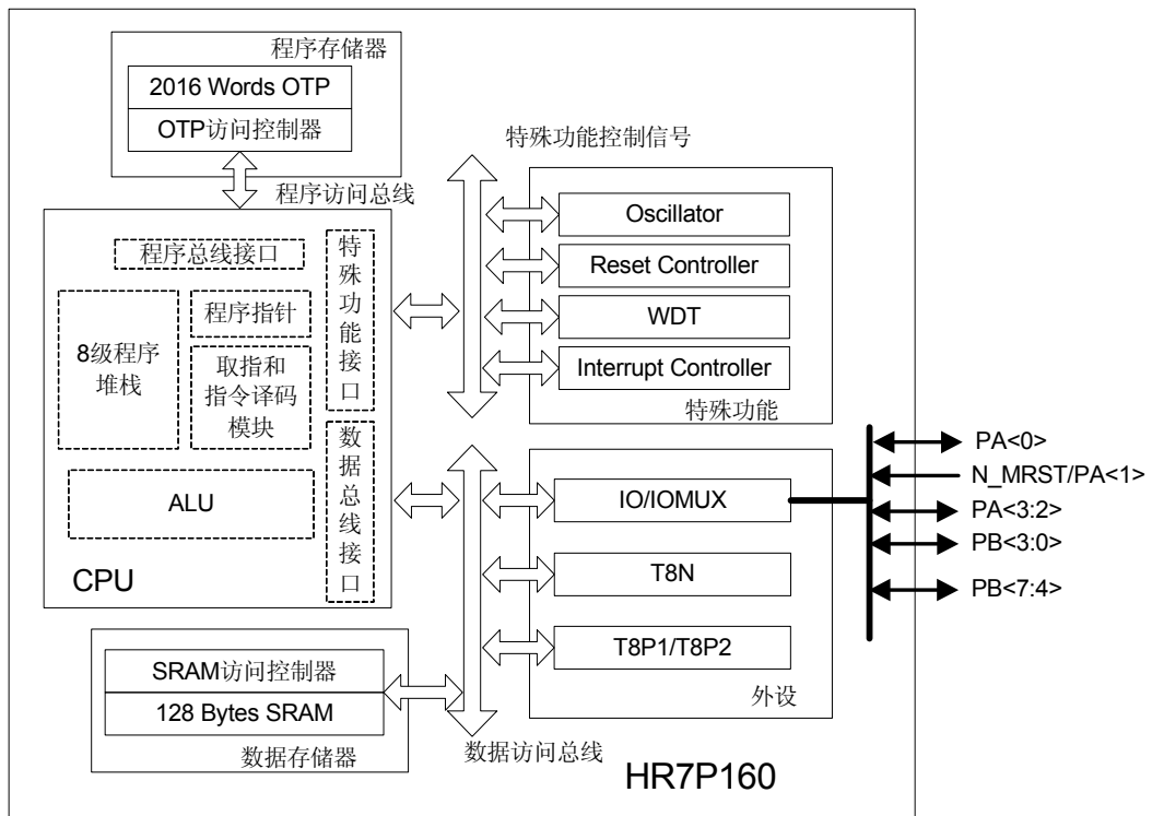
图 1-1 HR7P160 结构框图
