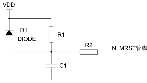
图 6-12 N_MRST 复位参考电路图 1
