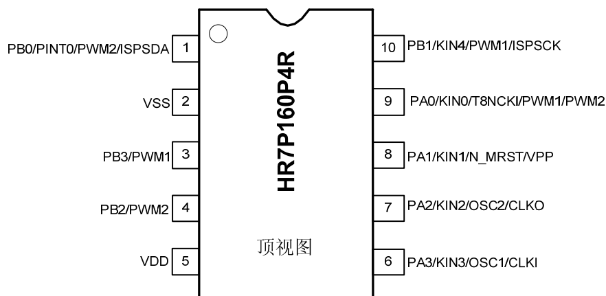
图 1-3 HR7P160P4R (SSOP10) 顶视图
