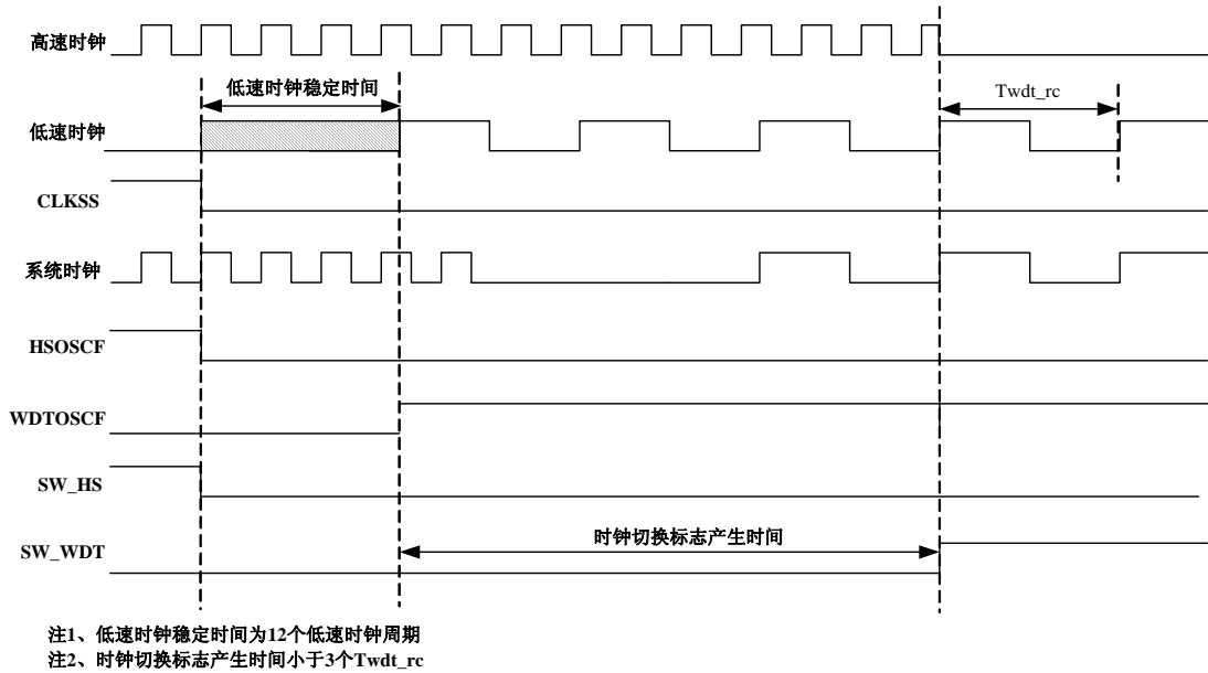
图 6-5 INTOSCH/HS/XT 时钟切换到 INTOSCL 时钟
