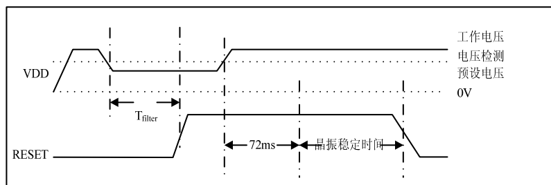
图 6-11 低电压复位时序示意图
