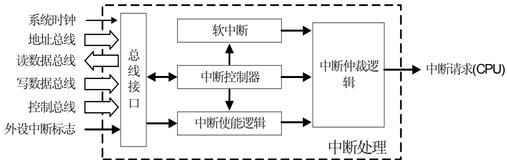
图 6-14 中断控制逻辑
