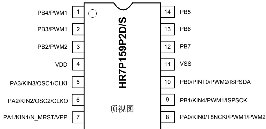
图 1-2 HR7P159P2D/S (DIP14/SOP14) 顶视图
