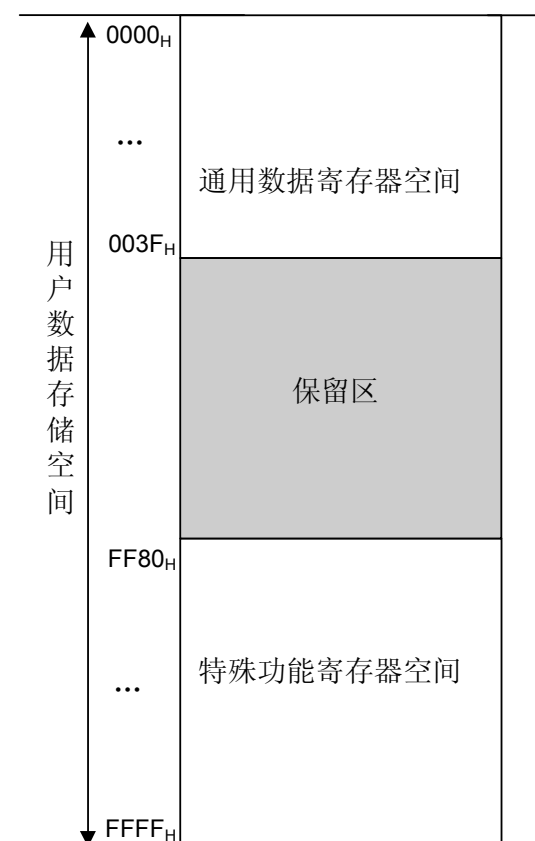
图 3-2 数据区地址映射示意图
