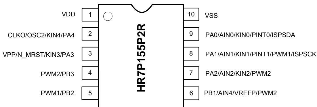
图 1-3 SSOP10 顶视图
