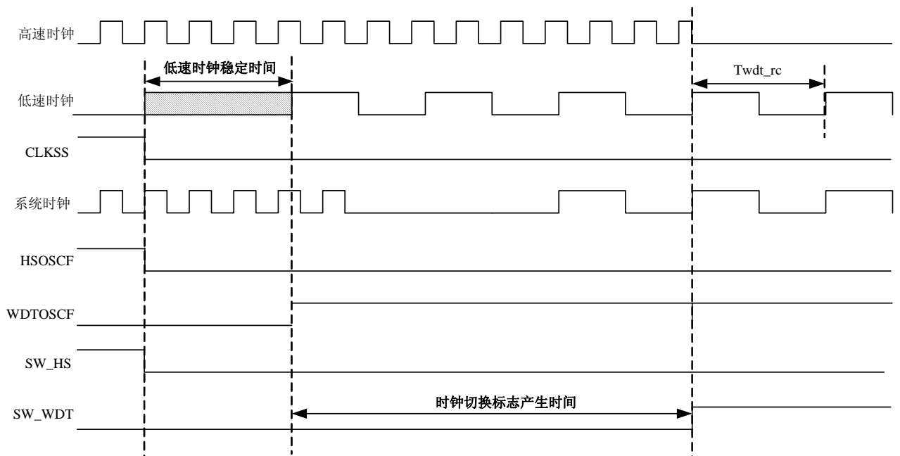
图 6-5 INTOSCL 时钟切换到 HS/XT/RC/INTOSCH 时钟时序图
