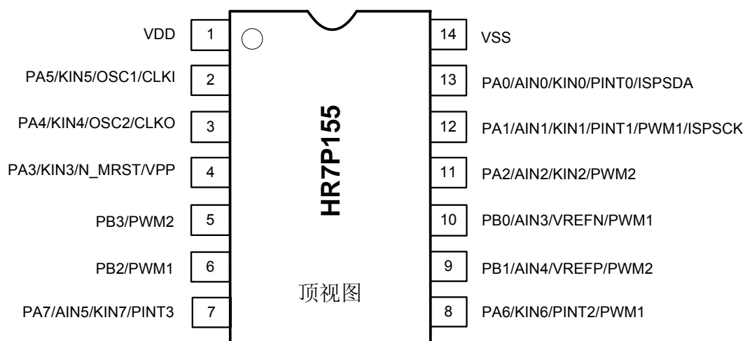
图 1-2 DIP14/SOP14 顶视图
