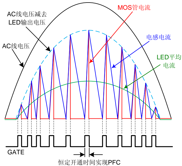
图2.功率因子校正示意图
