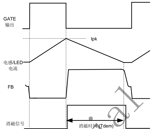
图3.芯片内部消磁检测控制
