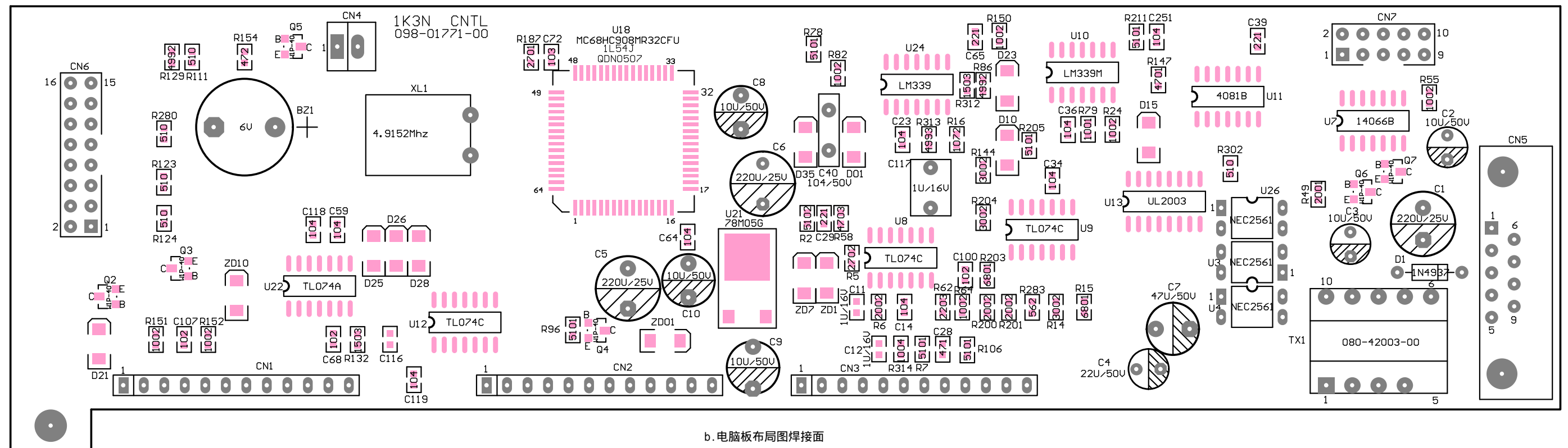
图7.10 SANTAK-1K3N型高频机电脑板布局图
