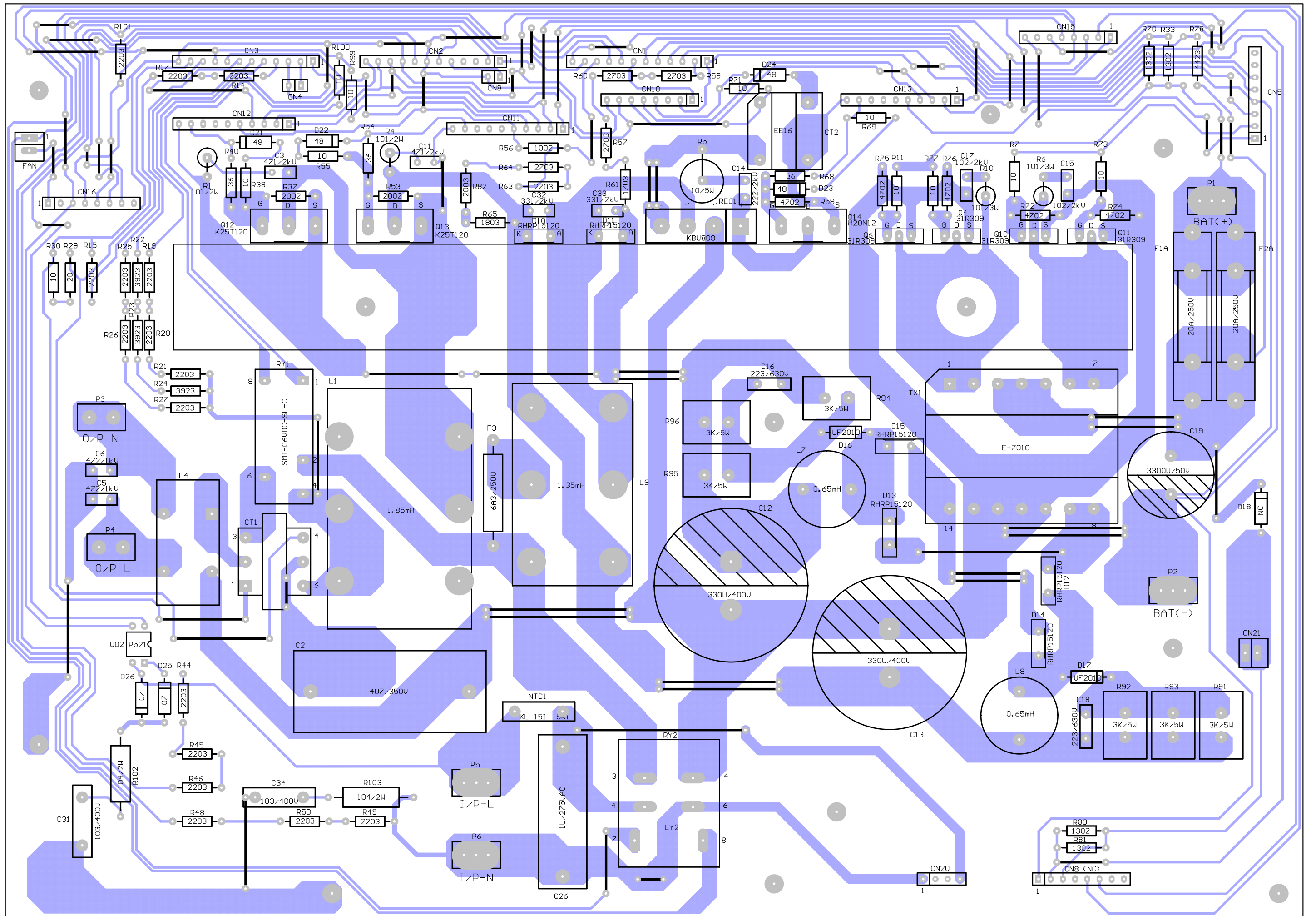
图7.3 SANTAK-1053型高频机主板印版图
