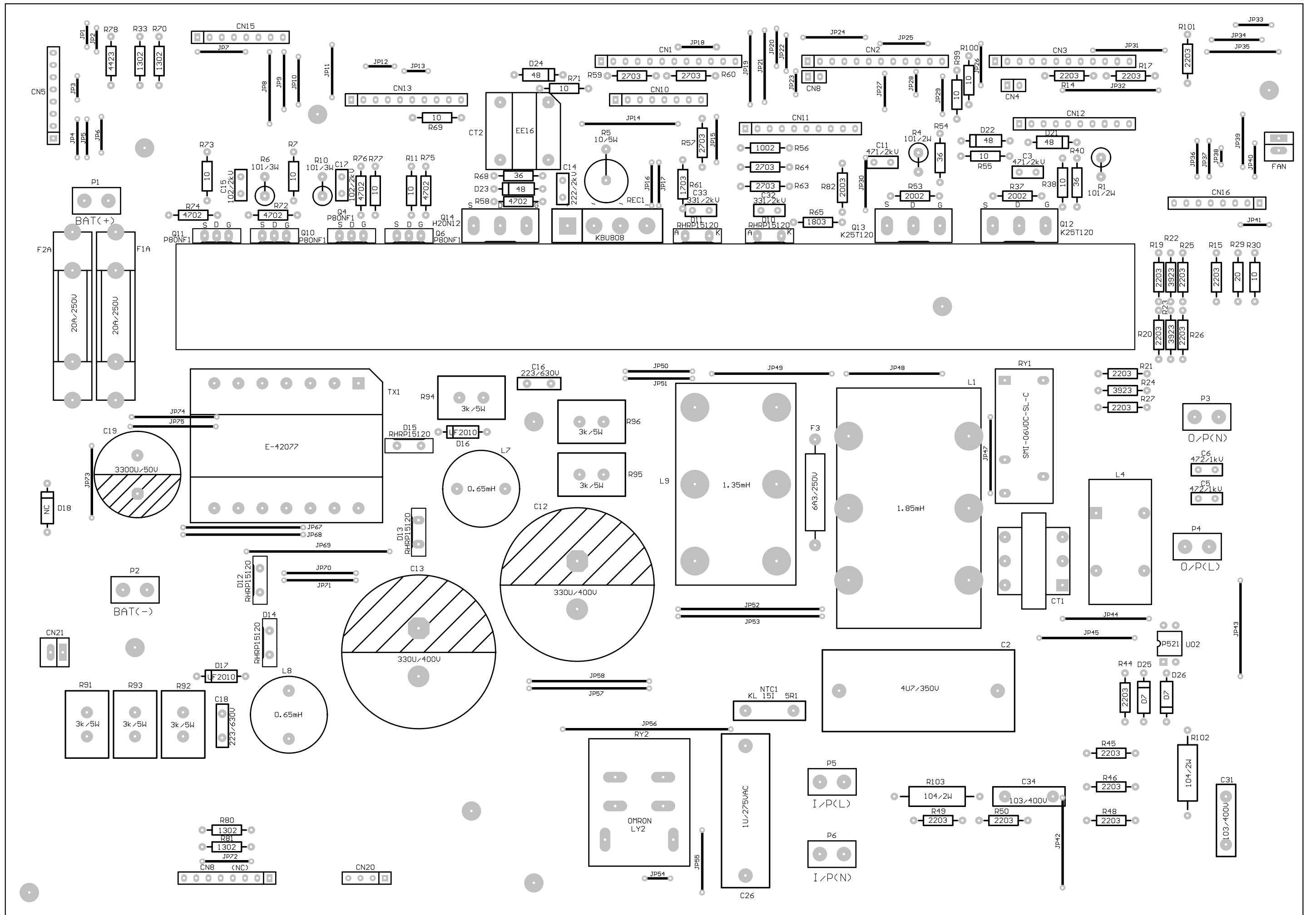
图7.2 SANTAK-1K3N型高频机主板布局图
