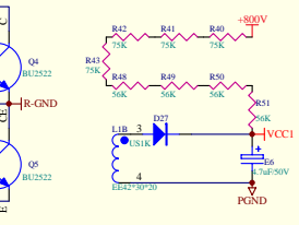
半桥功率电路
