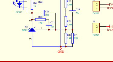
辅助供电测试
