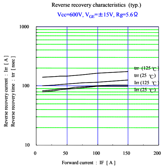
图 2-16 t_{rr} 、 I_{rr}-I_F 特性
