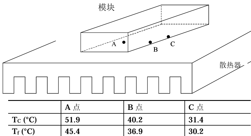
图 6-7 外壳温度测定实例
