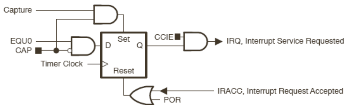
图 9-15 捕获比较 TBCCR0 中断标志
