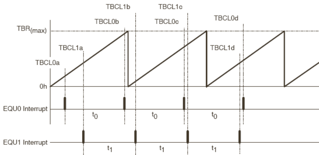
图 9-6. 连续模式时间间隔
