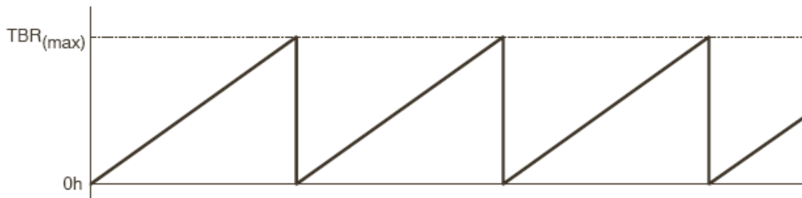
图 9-5. 连续模式标志位的设置
