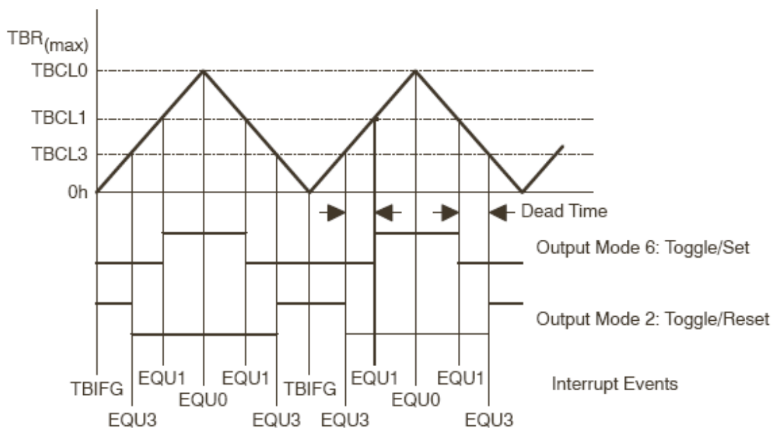
图 9-9. 增减模式的输出
