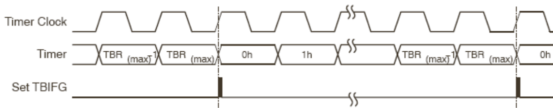
图 9-5. 连续模式标志位的设置
