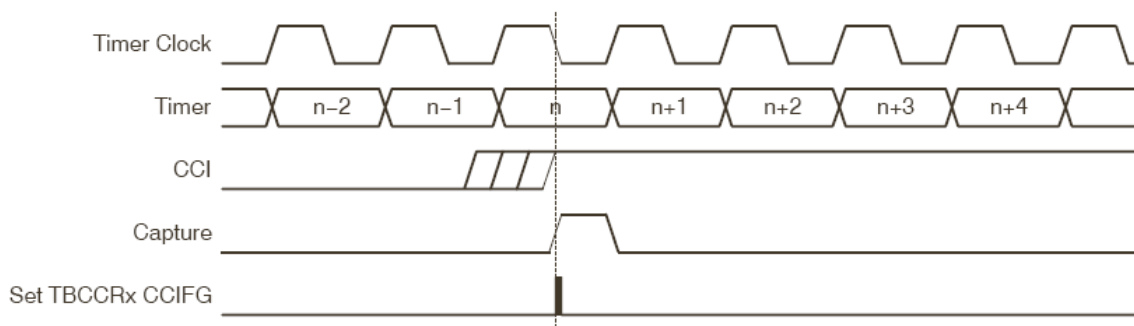
图 9-10. 捕获信号 (SCS=1)
