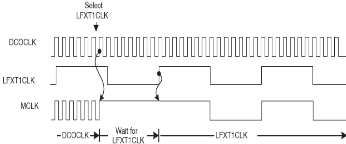
图 4-8 MCLK 的时钟源从 DCO 转换为 MCLK
