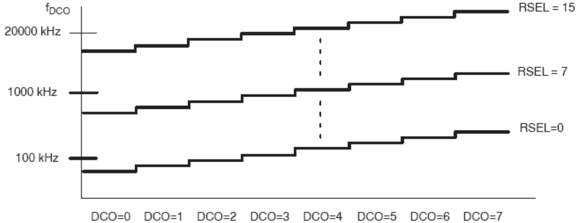
图4-5 典型DCOx的范围和RSELx步进
