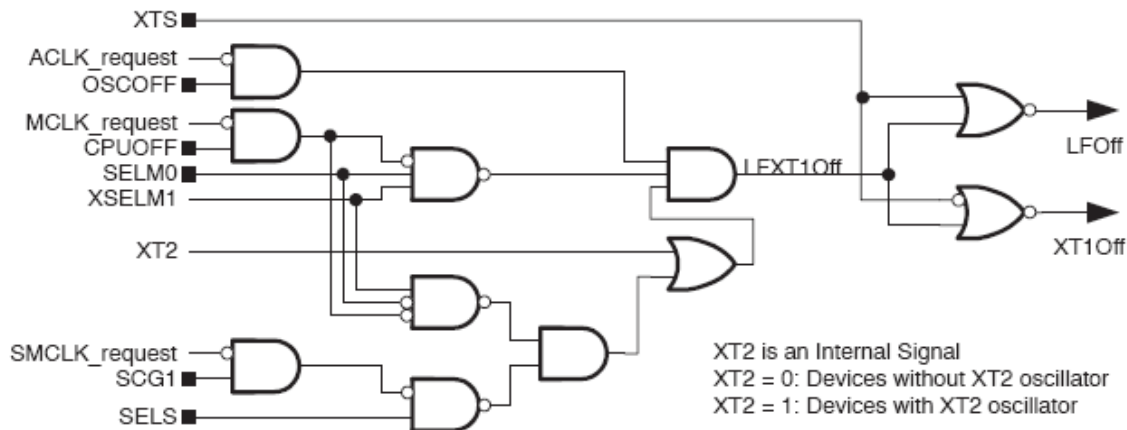
图4-2 LFXT1振荡器信号
