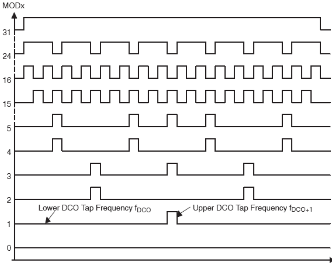
图4-6 调节器模式
