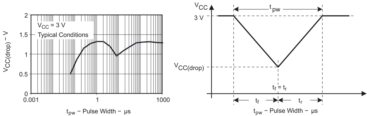
Figure 14. 具有一个三角形压降的 V_{CC(drop)} 电平用于生成一个上电复位 (POR) / 欠压信号
