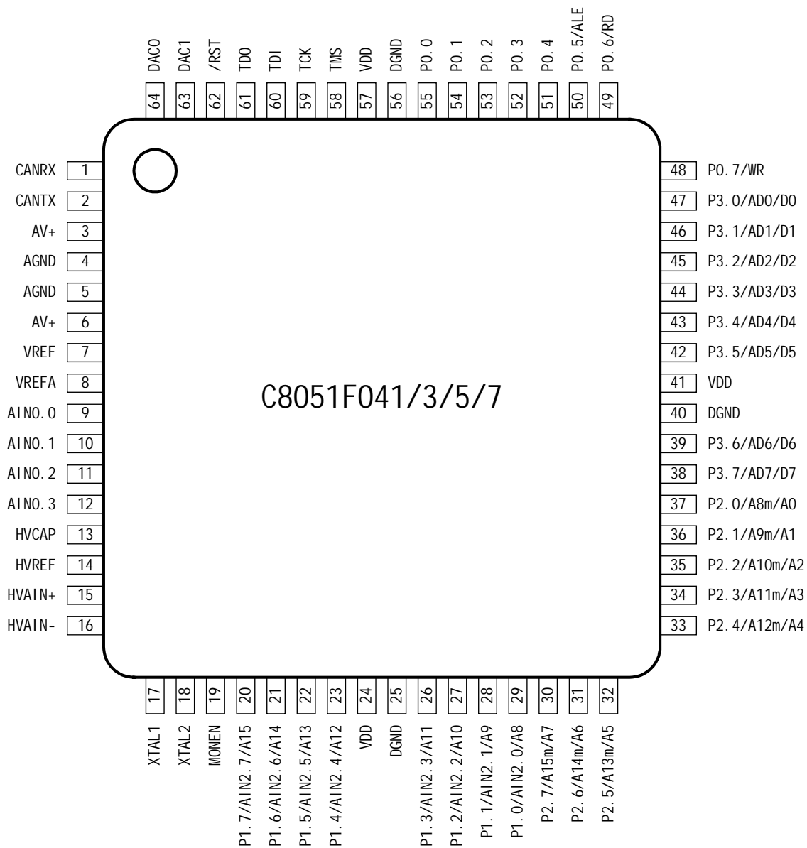
图 4.3 TQFP-64 引脚图
