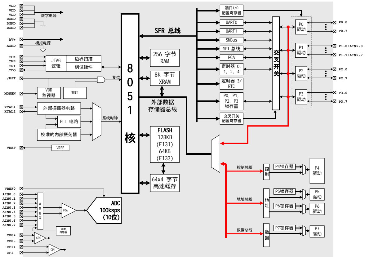
图 1.6 C8051F131/133 原理框图
