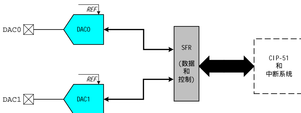
图1.15 DAC原理框图
