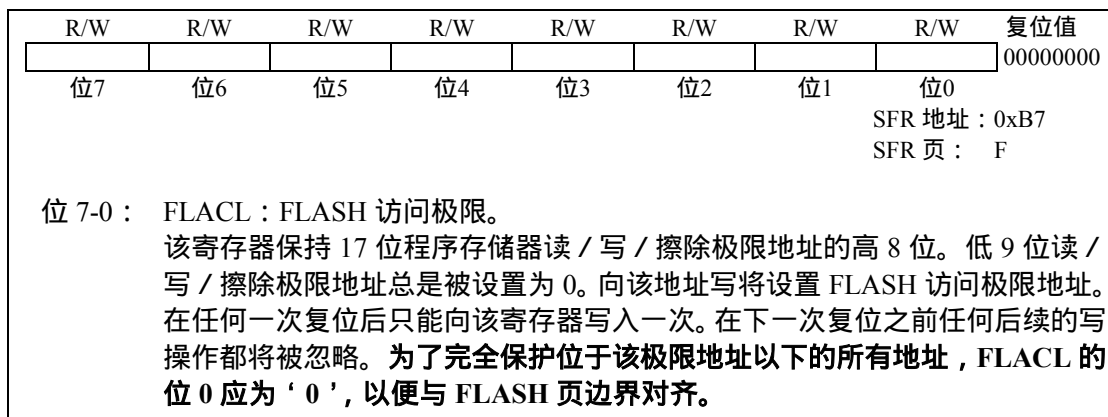
图 15.4 FLACL: FLASH 访问极限寄存器
