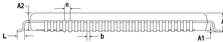
图 4.3 TQFP-100 封装图
