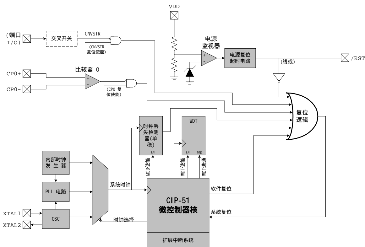
图 13.1 复位源框图
