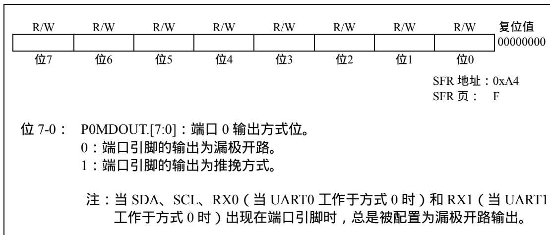
图 18.11 P0MDOUT：端口 0 输出方式寄存器
