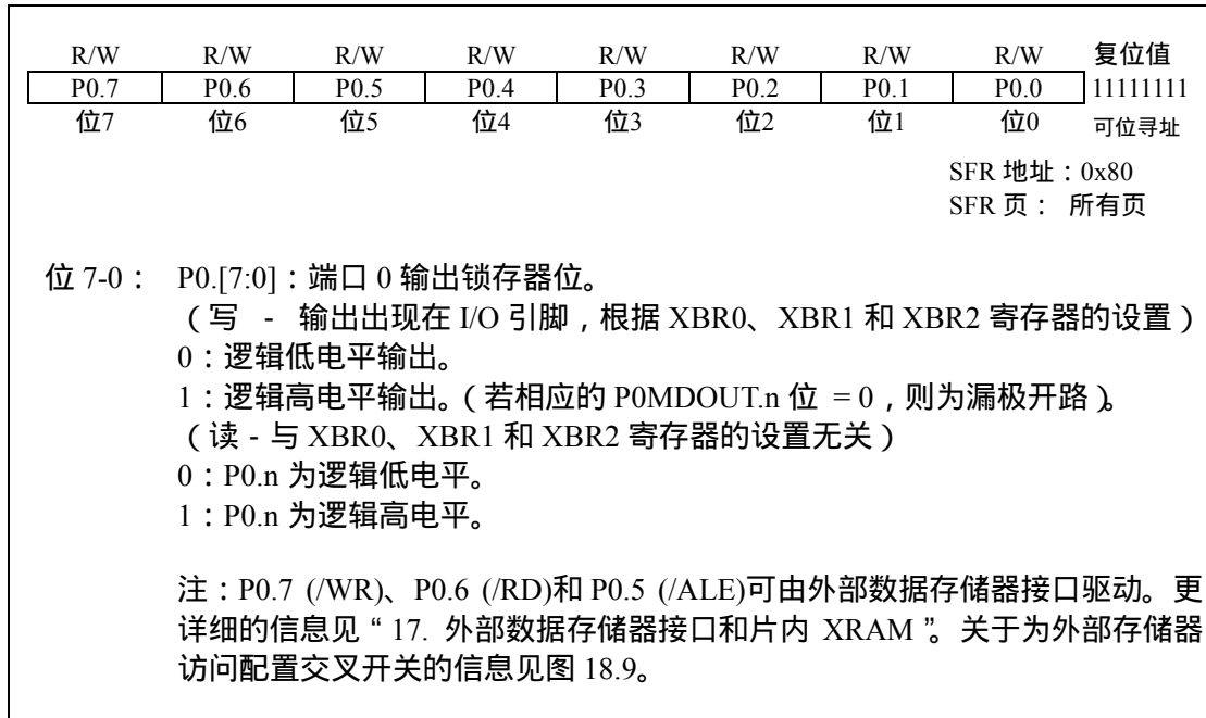
图 18.10 P0：端口 0 寄存器
