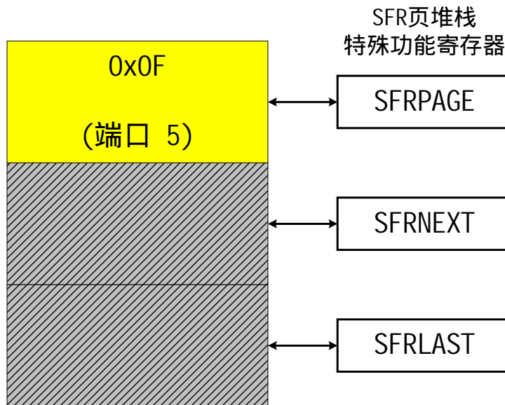
图 11.6 SFR 页堆栈：用 SFR 页 0x0F 访问端口 5
