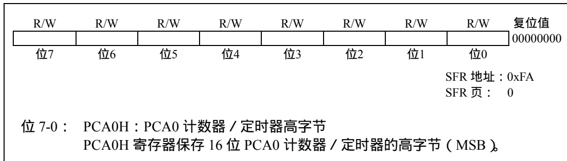
图 24.14 PCA0H：PCA0 计数器 / 定时器高字节
