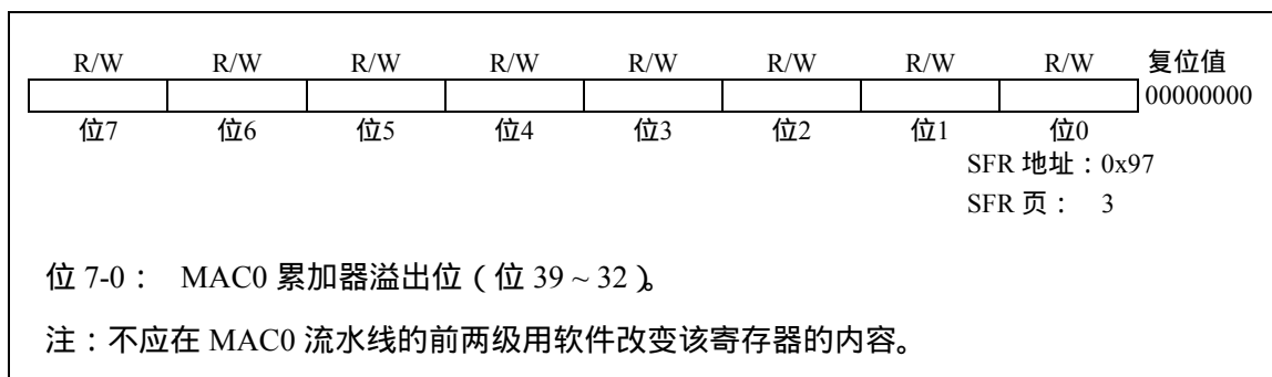
图 12.18 MAC0OVR：MAC0 累加器溢出寄存器
