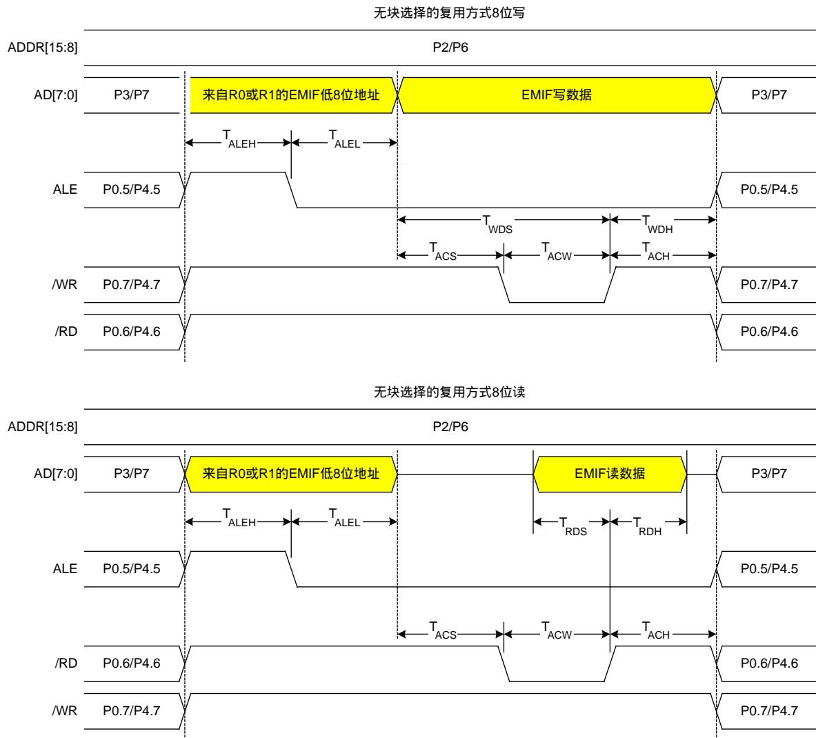
图 17.11 无块选择的复用方式 8 位 MOVX 时序
