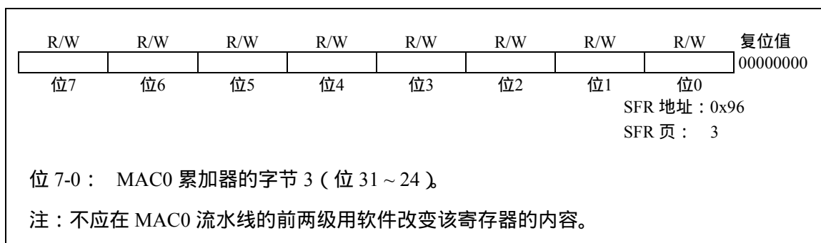
图 12.14 MAC0ACC3：MAC0 累加器字节 3 寄存器
